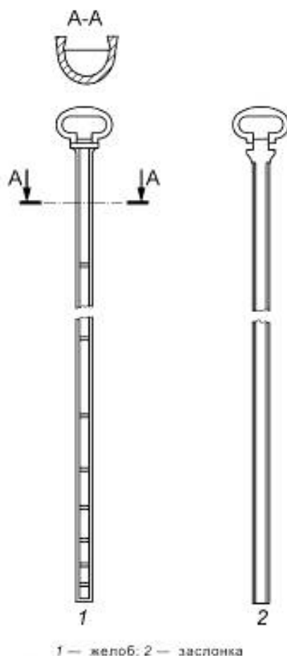
Рисунок 1 — Желобчатый пробоотборник для взятия проб жидкостей
