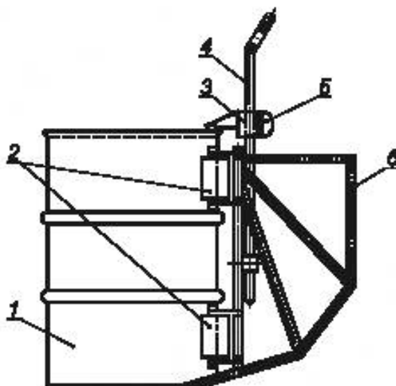
ДБ.5 Устройство для перемешивания с применением рамы (рисунок ДБ.5)
