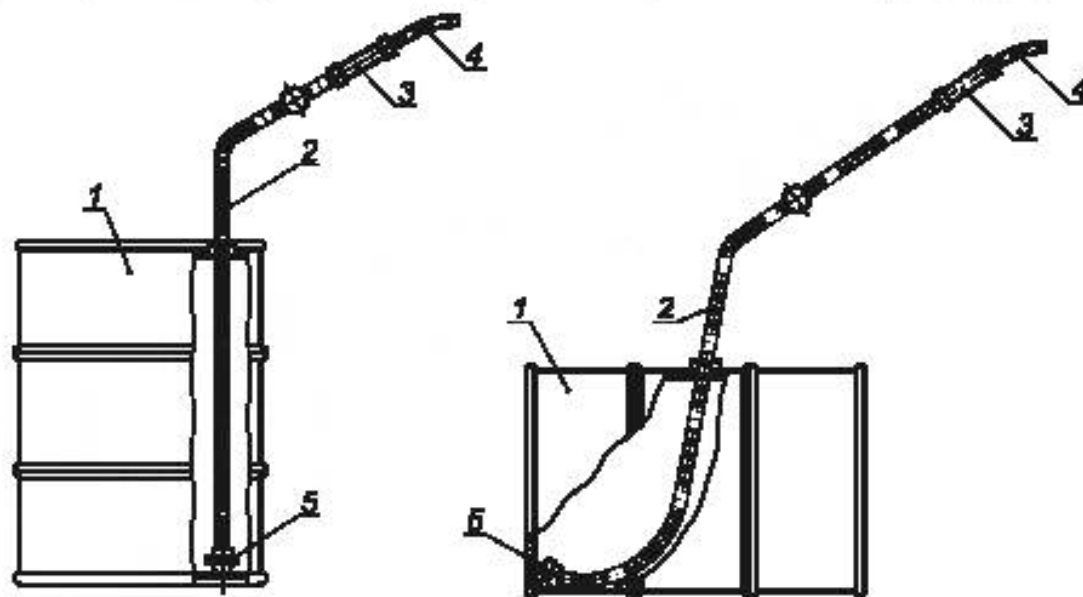
ДБ.4 Устройство для перемешивания с применением труб и наконечников (рисунок ДБ.4)
