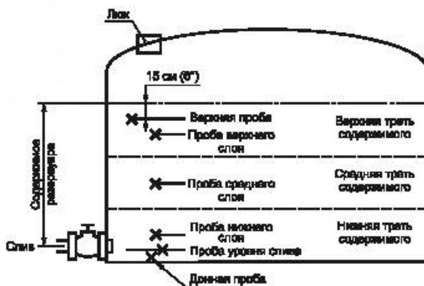
Рисунок 11 — Отбор проб из больших емкостей
