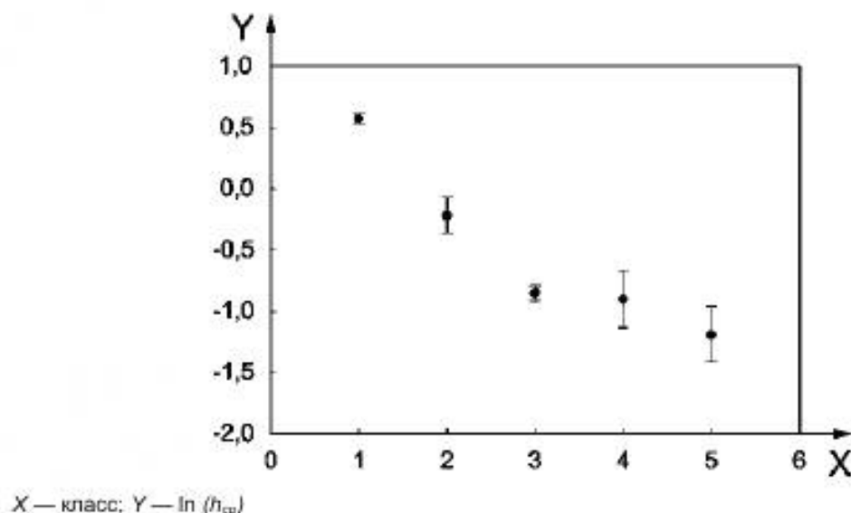
Рисунок В. 6 — Соотношение между классом и преобразованным h_{cp}
