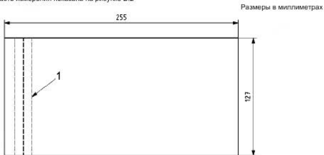
Рисунок В.2 — Область измерения реплики помятости
