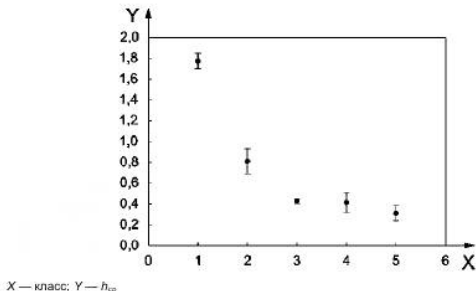
Рисунок В.5 — Соотношение между классом и исходным h_{cp}
