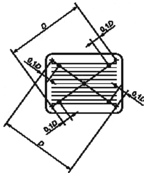
Рисунок 3 — Точки измерения для ЭЛТ-дисплеев
