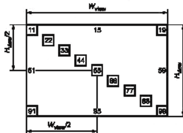
Рисунок 4 — Точки измерения для ЖК-дисплеев
