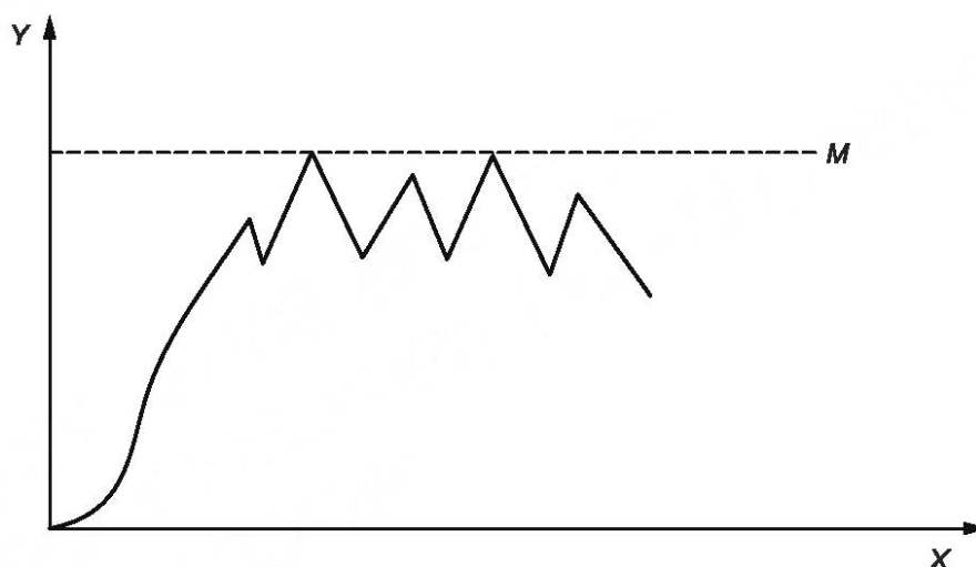
а) Типовая кривая раздира
