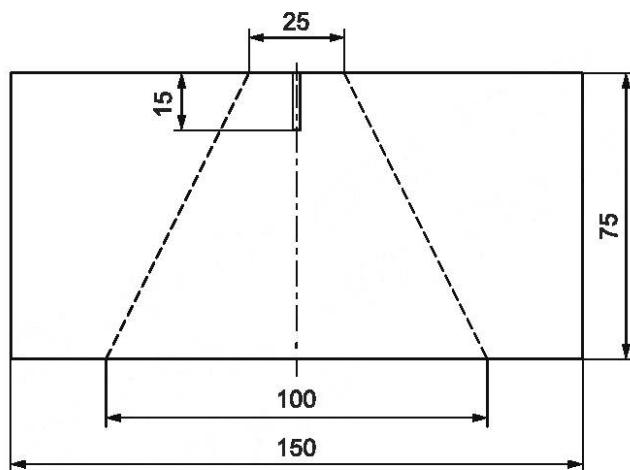
Рисунок 2 — Испытываемая проба с размеченной равнобедренной трапецией
