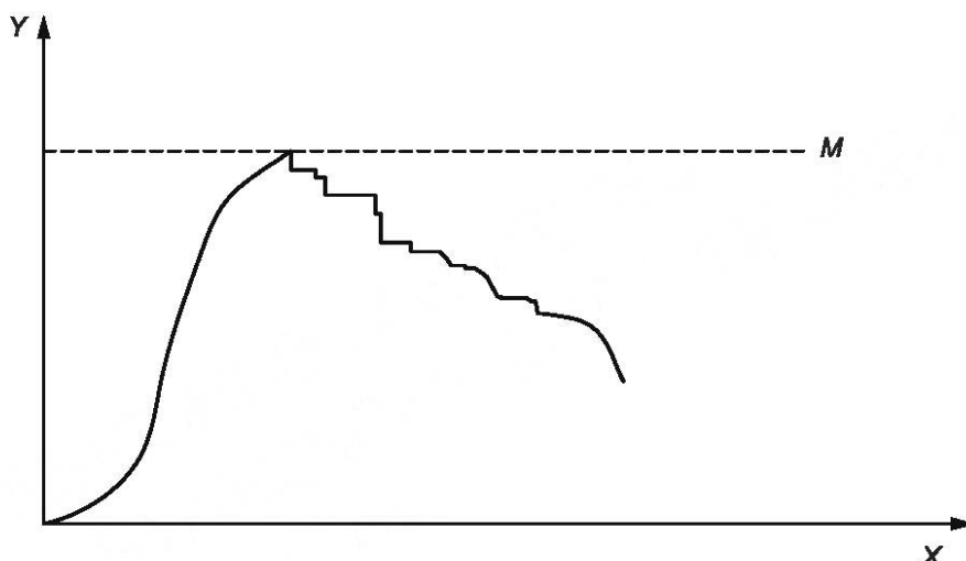
b) Другая типовая кривая раздира
