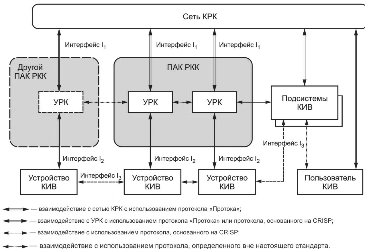
Рисунок 1 — Интерфейсы ПАК РКК и взаимодействующих с ним элементов на прикладном уровне
