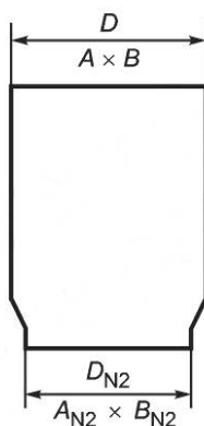
b) Цилиндрические банки с зауженной горловиной (донышком)
