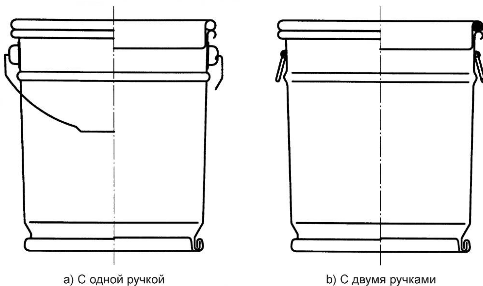
Рисунок 2— Ведро
