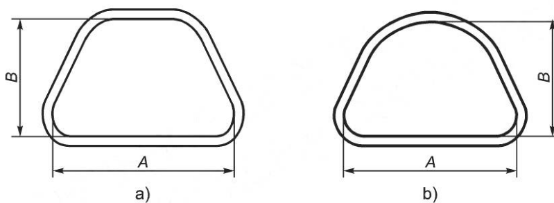
Рисунок 13 — Трапецевидные банки
