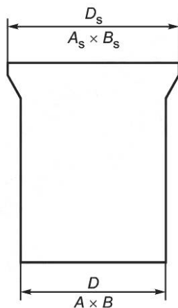
d) Цилиндрические банки с расширенной горловиной
