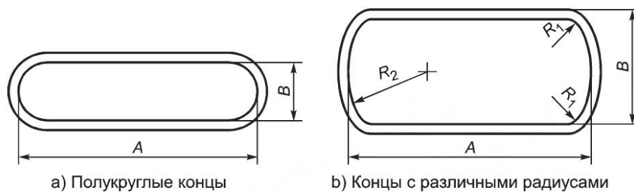
Рисунок 11 — Закругленные банки
