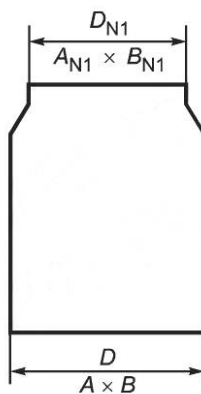
c) Цилиндрические банки с зауженной горловиной (крышкой)
