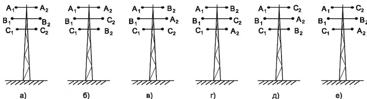
а) осевая симметрия фаз; б), в) — перемена мест двух фаз; г), д) — круговая перестановка фаз одной цепи; е) — центральная симметрия фаз (угол сдвига фаз \varphi_{\text{ф}} : А = 120^\circ , В = 0^\circ , С = -120^\circ )
