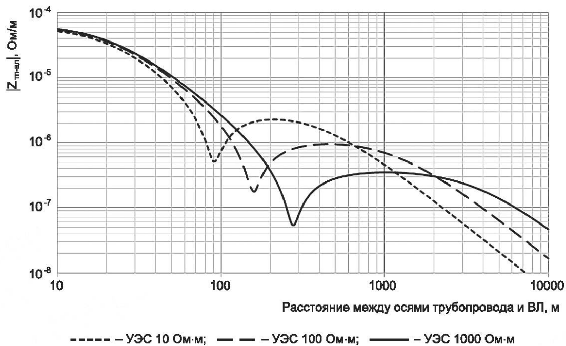
Рисунок Е.8 — Взаимное магнитное сопротивление между трубопроводом и ВЛ на опоре УЗ30-2 в нормальном режиме работы при различных УЭС грунта
