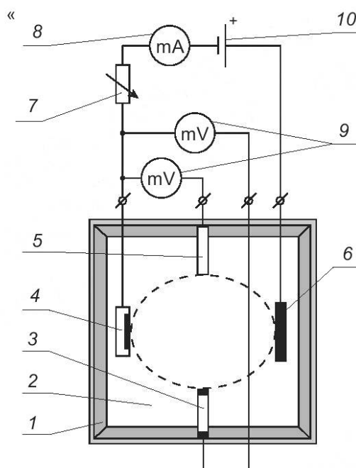
1 — диэлектрическая емкость; 2 — испытательная среда; 3 — испытуемый ЭС; 4 — вспомогательный электрод (катод); 5 — ЛЭС; 6 — рабочий электрод (анод); 7 — регулирующий резистор; 8 — миллиамперметр; 9 — милливольтметр; 10 — источник тока».
