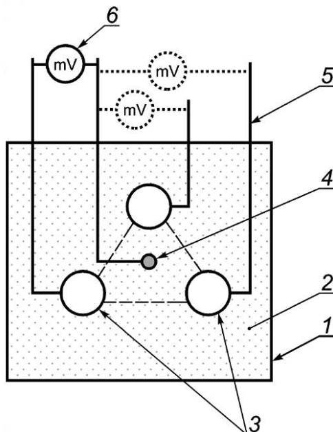
1 — диэлектрический контейнер; 2 — испытательная среда; 3 — испытуемые ЭС; 4 — лабораторный (контрольный) электрод; 5 — кабельный вывод от электрода; 6 — милливольтметр
