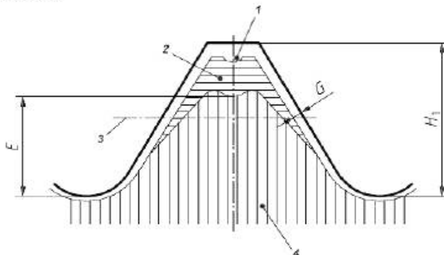
1 – зона полного обезуглероживания; 2 – зона частичного обезуглероживания или ферритного обезуглероживания; 3 – линия среднего диаметра резьбы; 4 – зона основного металла; E – высота необезуглероженой зоны резьбы; G – глубина полного обезуглероживания в резьбе; H_1 – высота наружной резьбы полного профиля
