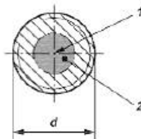
1 – ось крепежного изделия; 2 – область половины радиуса сечения (радиус 0,25d )
