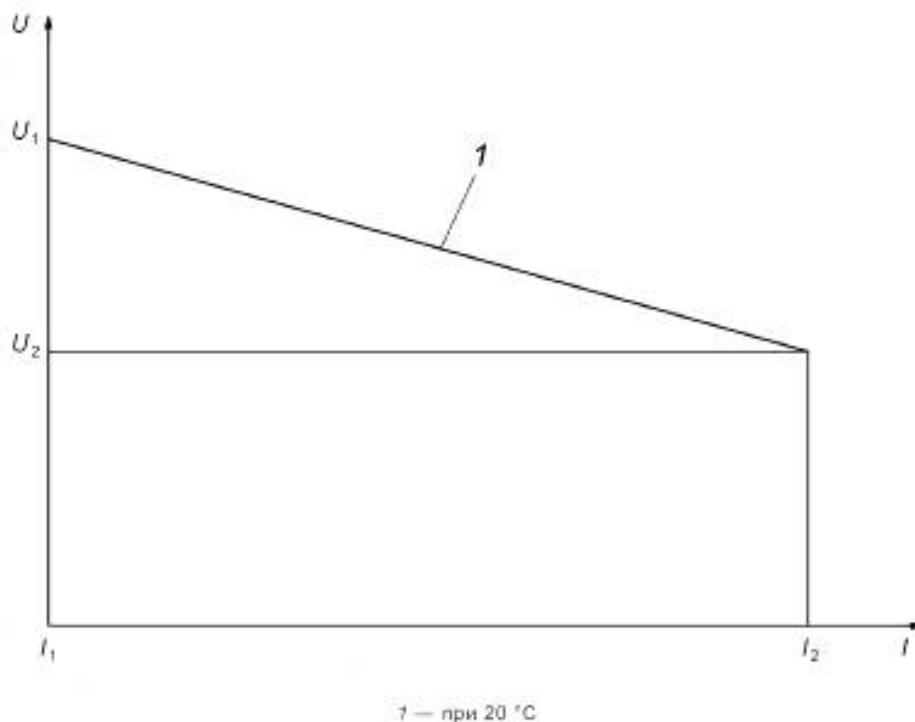
Рисунок 1 — Вольтамперная характеристика источника питания стартера
