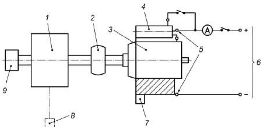
1 — тормоз переменной нагрузки; 2 — муфта; 3 — стартер; 4 — соленоид (тянущее реле); 5 — выводы стартера; 6 — питание стартера; 7, 8 — точки измерения крутящего момента; 9 — измерение частоты вращения
