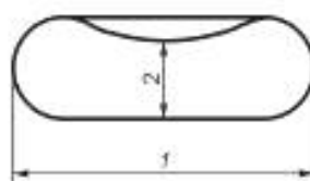
Рисунок 12 — Линейные измерения подследников
