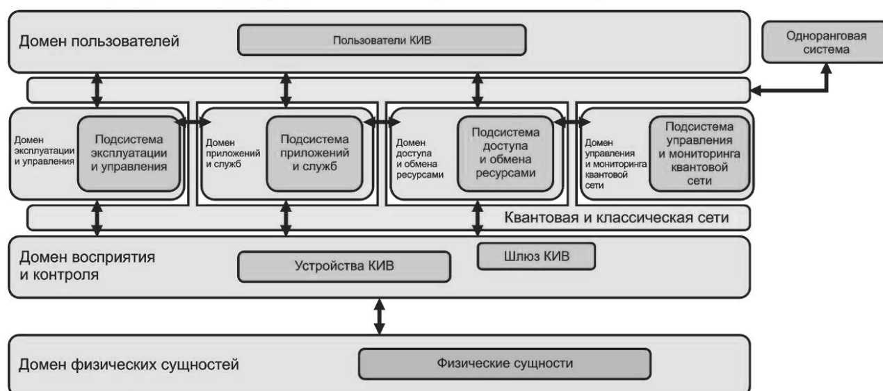
Рисунок 4 — Сопоставление типовых моделей КИВ на основе сущностей и на основе доменов
