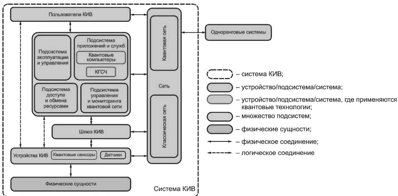
Рисунок 2 — Типовая модель КИВ на основе сущностей
