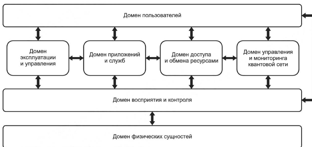
Рисунок 3 — Типовая модель КИВ на основе доменов
