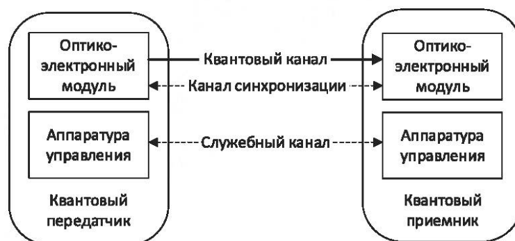
Рисунок 1 — Типовая схема системы квантовой коммуникации
