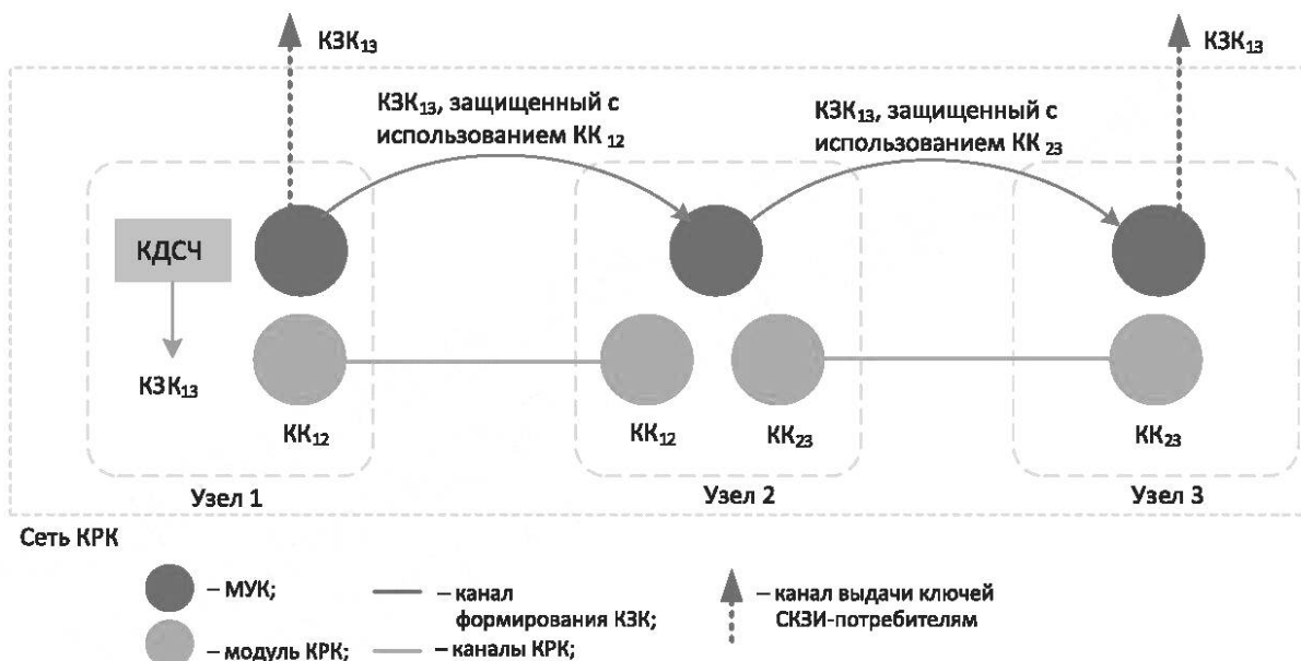
Рисунок 8 — Пример формирования КЗК в сети КРК с использованием КДСЧ
