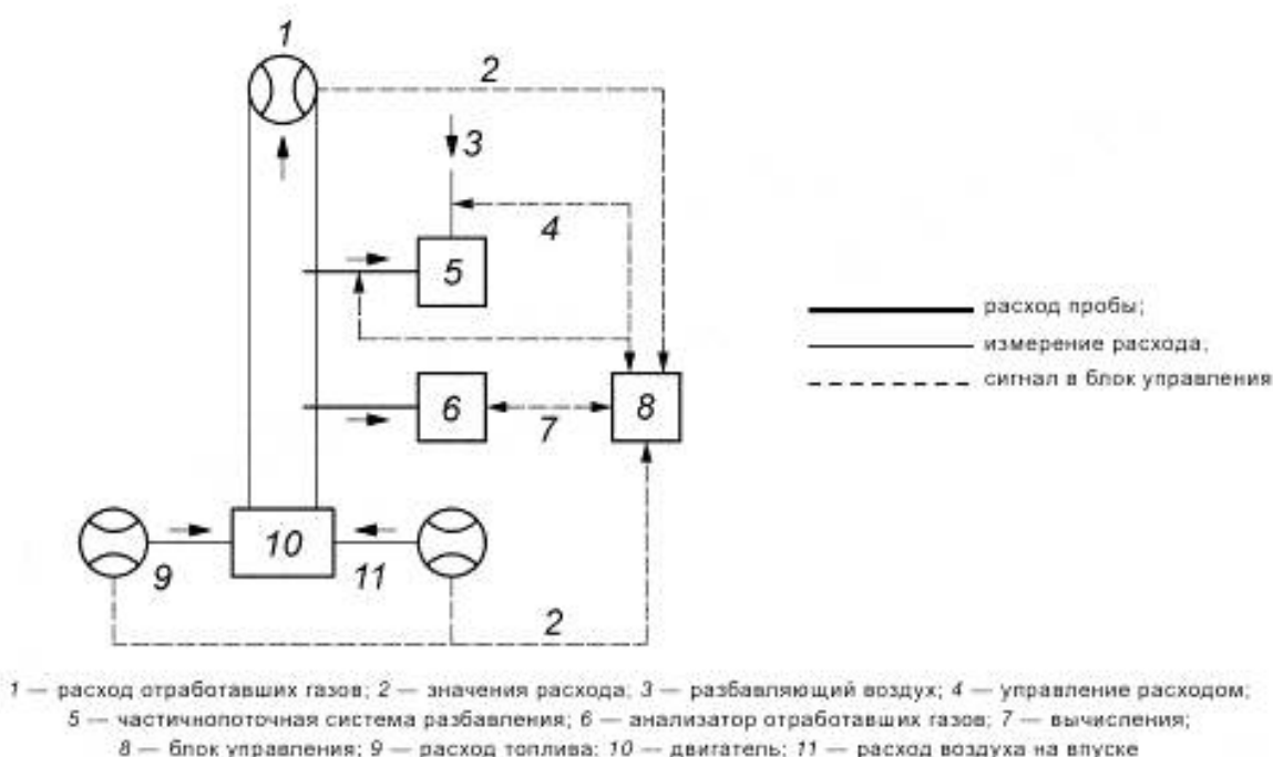
Рисунок 2 — Схема измерений в полнопоточной/частичнопоточной системах разбавления
