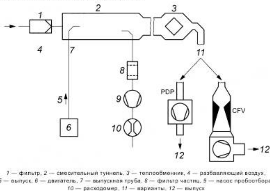
Рисунок 3 — Схема полнопоточной системы разбавления CVS
