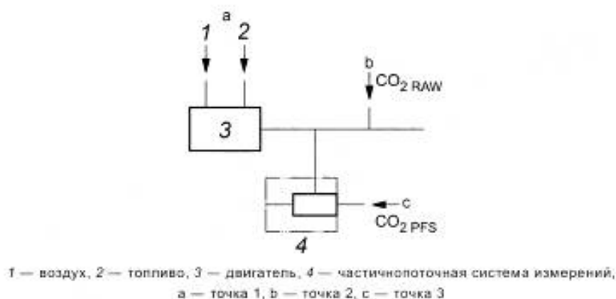
Рисунок D.1 — Точки измерения расхода углерода
