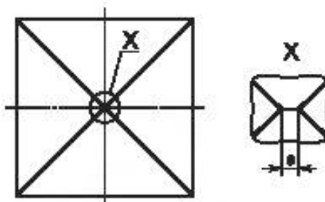
Рисунок 2 — Угол алмазной пирамиды Виккерса
