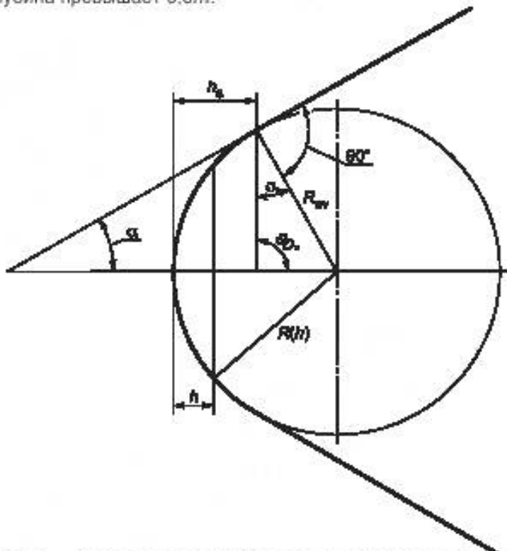
Рисунок 6 — Иллюстрация параметров сферических наконечников
