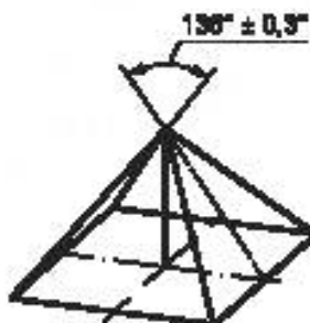
Рисунок 2 — Угол алмазной пирамиды Виккерса
