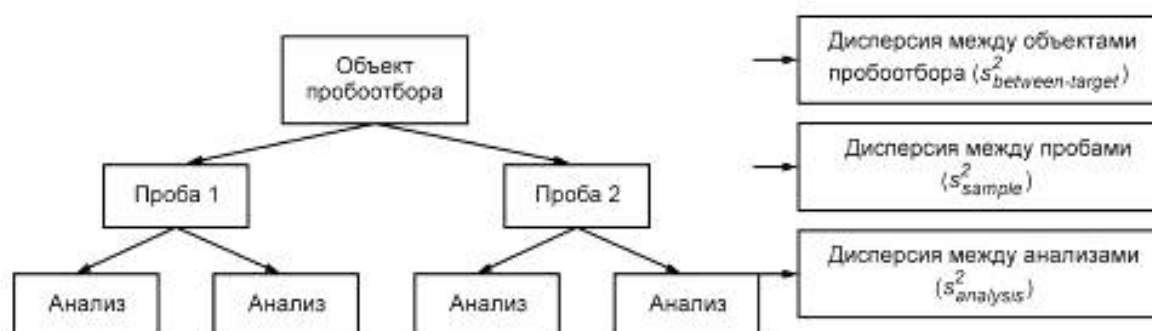
Рисунок 2 — Сбалансированный план пробоотбора
