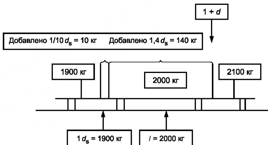
Рисунок 1 — Пример испытания весов с d_s = 100 кг на реагирование
