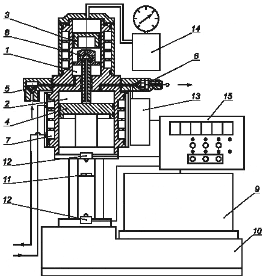
1 — проботборная камера; 2 — измерительная камера; 3, 4 — поршни; 5 — входной клапан; 6 — выходной клапан; 7 — термостатирующая рубашка; 8 — впрыскной клапан; 9 — двигатель; 10 — редуктор; 11 — визир; 12 — микровыключатели; 13 — датчик давления; 14 — подпорная газовая камера; 15 — блок управления (панель приборов)
