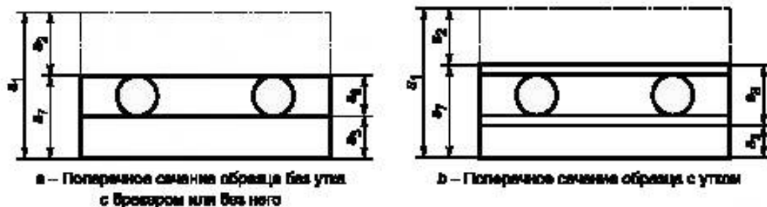
Рисунок 3 — Образцы для метода A1
