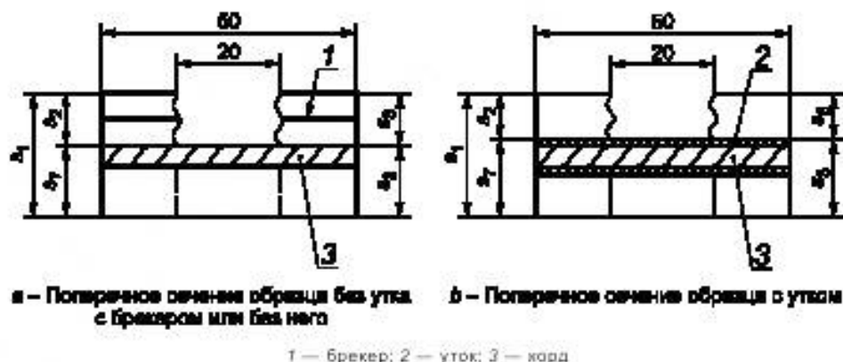
Рисунок 4 — Испытуемые образцы для метода A2
