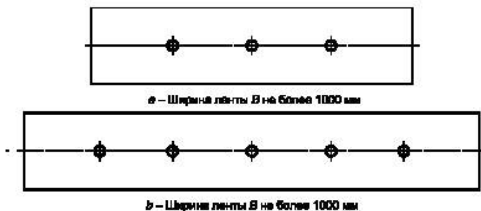
Рисунок 1 — Расположение точек измерения
