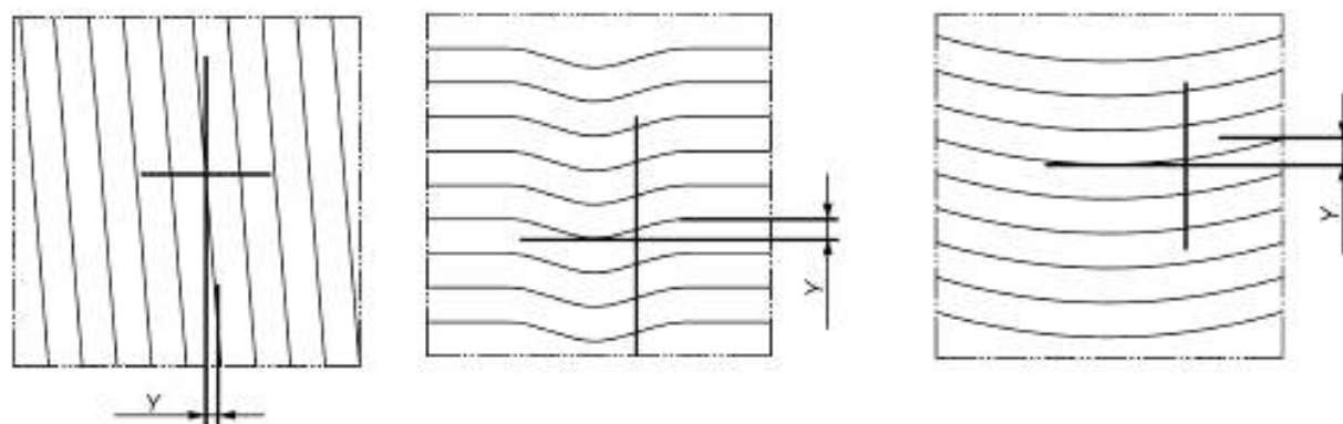
Рисунок 1 — Примеры смещения проволоки
