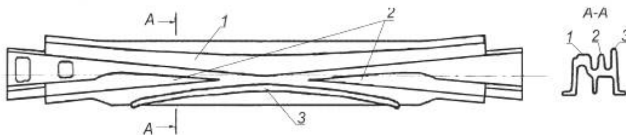
Рисунок 3.8 — Тупая цельнолитая крестовина (отливка)
