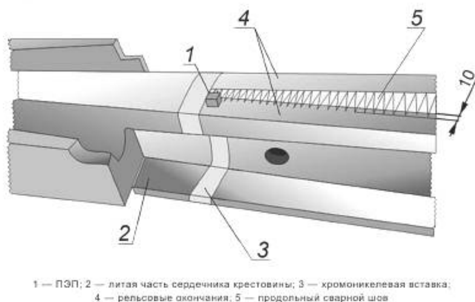
Рисунок В.2 — УЗК продольного сварного шва сварки рельсовых окончаний в области головки
