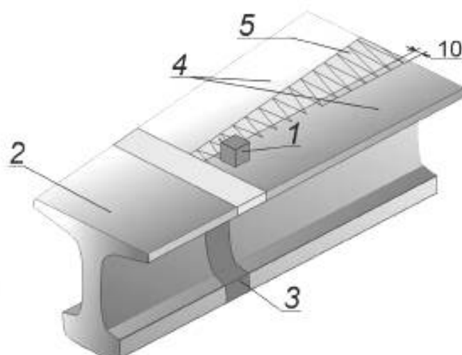
1 — ПЗП; 2 — литая часть сердечника крестовины; 3 — хромоникелевая вставка; 4 — рельсовые окончания; 5 — продольный сварной шов
