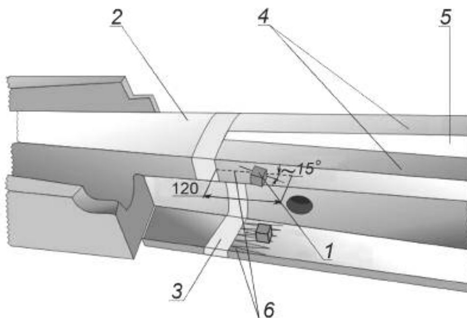
1 — ПЗП; 2 — литая часть сердечника крестовины; 3 — хромоникелевая вставка; 4 — рельсовые окончания; 5 — продольный сварной шов; 6 — траектории перемещения ПЗП
