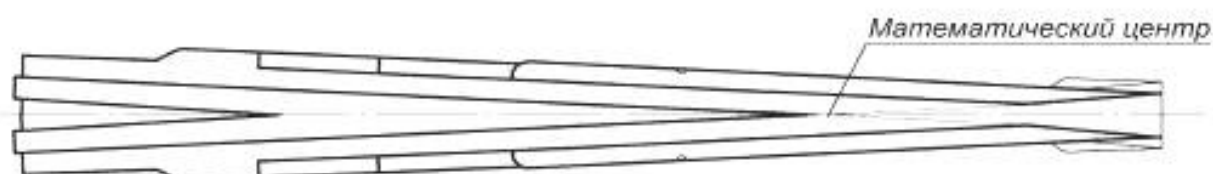
Рисунок 3.9 — Положение МЦК литого сердечника сборной крестовины
