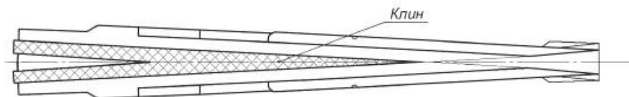
Рисунок 3.6 — Клин литого сердечника сборной крестовины
