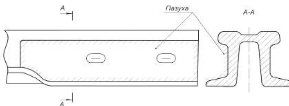
Рисунок 3.11 — Пазуха литого сердечника сборной крестовины
