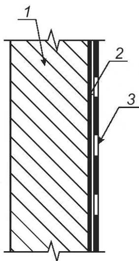
Рисунок А.2 — Сплошная бесшовная гидроизоляция стен
