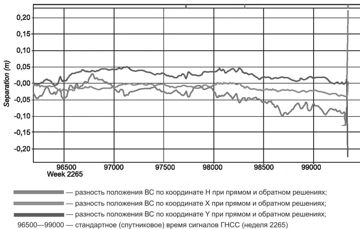
Рисунок Б.1 — Пример графиков обработки данных траектории полета воздушного судна. Разность координат прямого и обратного решений (м)
