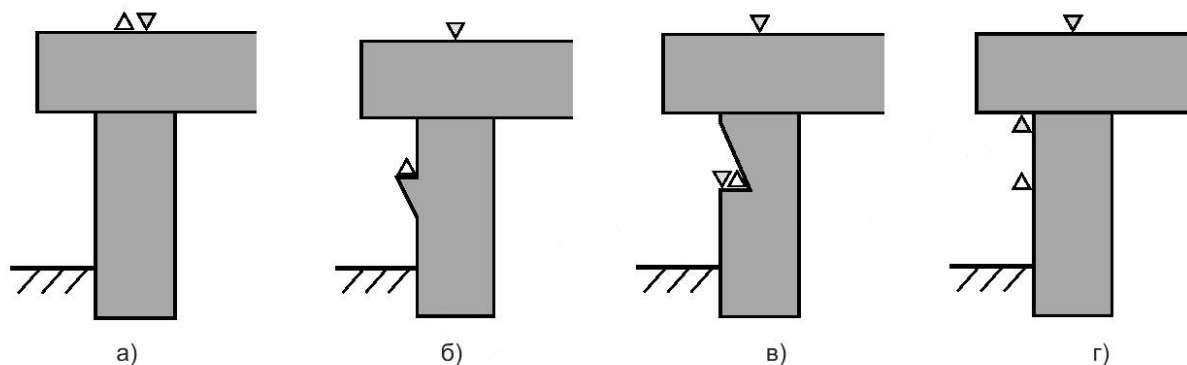
Рисунок 2 — Схемы взаимного расположения источника и приемника при обследовании сваи в составе ростверка
