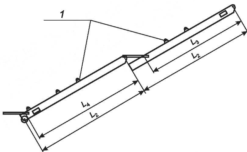
1 — промежуточные точки крепления; L_1 — номинальная длина: L_1 = L_3 + L_4 ; L_2 — конструктивная длина для каждого отдельного марша трапа
