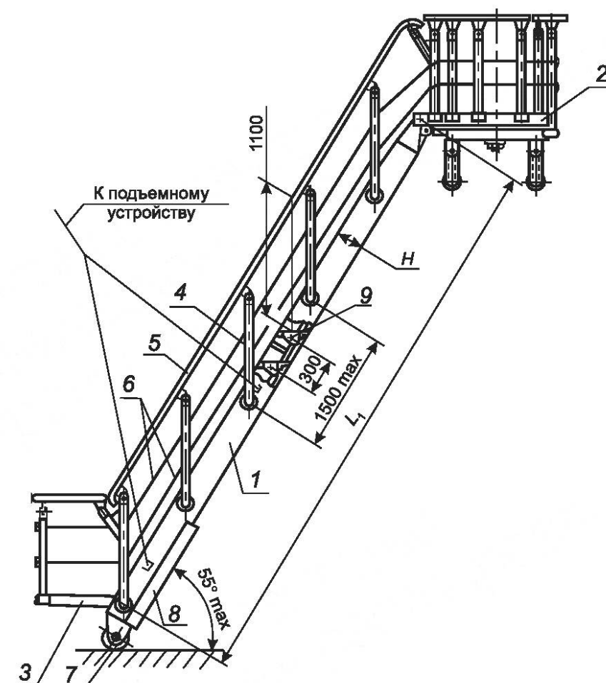
1 — тетива марша; 2 — верхняя поворотная площадка; 3 — нижняя площадка; 4 — леерная стойка; 5 — поручень; 6 — леер; 7 — опорный каток; 8 — привальный брус; 9 — поворотные ступени; L_1 — номинальная длина; H — высота тетивы марша
