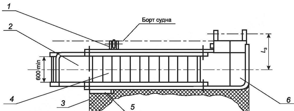
1 — бортовой каток; 2 — нижняя площадка; 3 — предохранительная сетка; 4 — ступени; 5 — привальный брус; 6 — верхняя стационарная площадка; L_3 — расстояние до осей крепления
