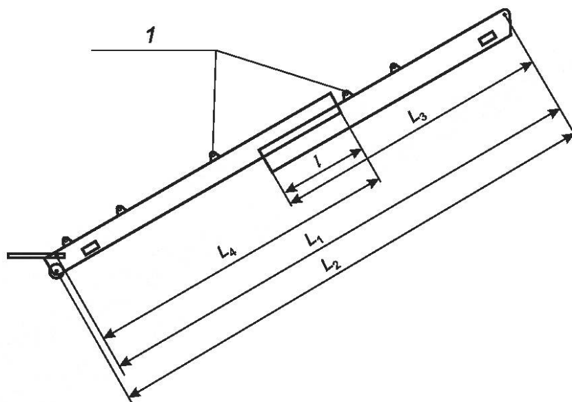
Рисунок 7 — Телескопический трап
