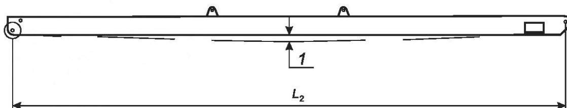
Рисунок 10 — Метод испытания для каждого марша
