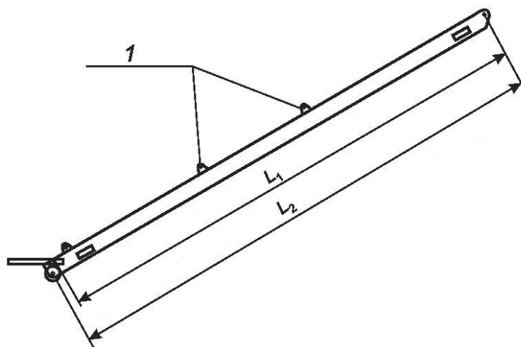
1 — промежуточные точки крепления; L_1 — номинальная длина; L_2 — конструктивная длина
