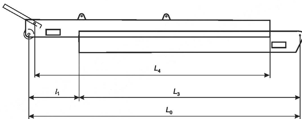
Рисунок 7 — Телескопический трап
