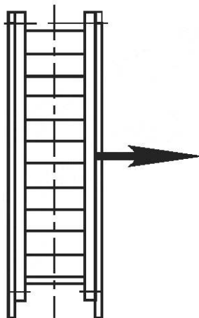
Рисунок 11 — Схема испытания поручней трапа на прочность
