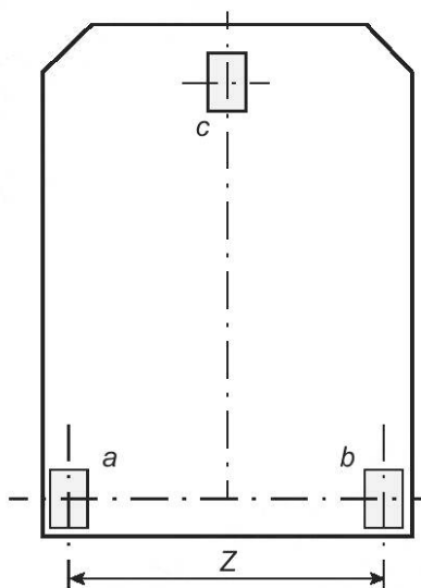
Рисунок 1 — Колея (ширина колеи)
