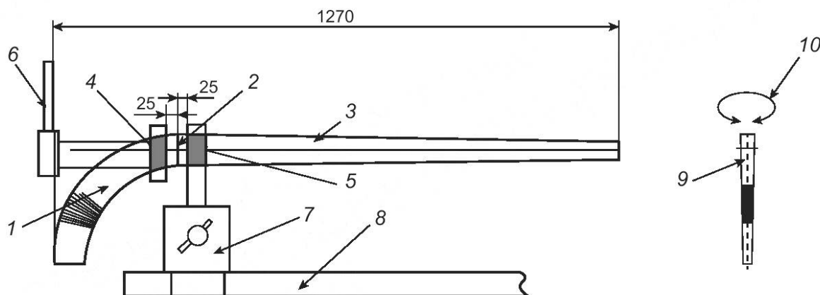
1 — крюк; 2 — место сопряжения крюка и ручки; 3 — рукоятка клюшки; 4 — зона фиксации крюка при проведении испытаний тисками динамометрического ключа; 5 — зона фиксации ручки тисками; 6 — динамометрический ключ; 7 — тиски; 8 — монтажный стол; 9 — ось клюшки; 10 — момент скручивания
