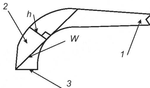
Рисунок 2 — Схема определения радиуса загиба крюка клюшки
