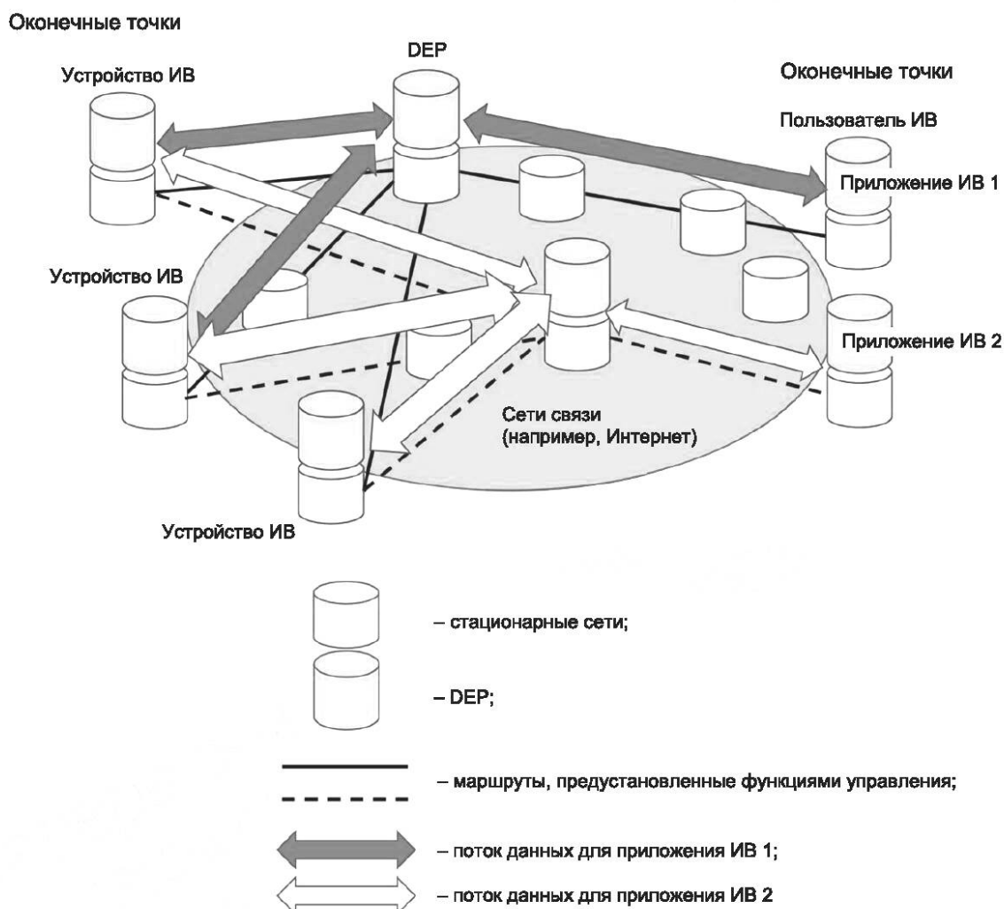
Рисунок 18 — Операции контроля информации с использованием DEP
