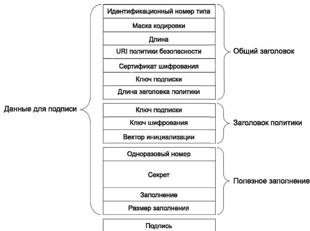
Рисунок 39 — Разбивка зашифрованного секрета
