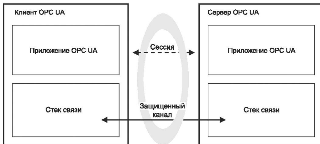
Рисунок 13 — Защищенный канал и службы сессии
