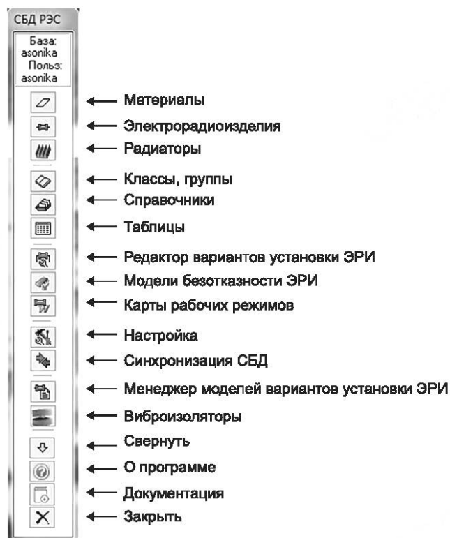
Рисунок А.1 — Главное окно подсистемы АСНИКА-БД
