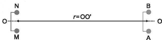
Рисунок 5 — Схема дипольной экваториальной установки профилирования
