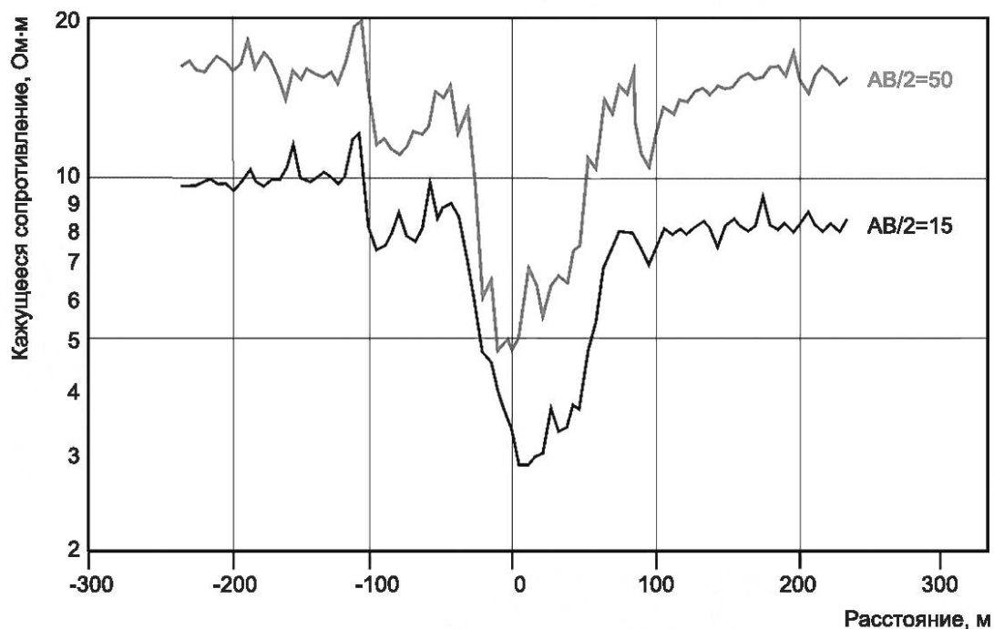
Рисунок Б.1 — Графики КС для двух действующих разносов ЭП
