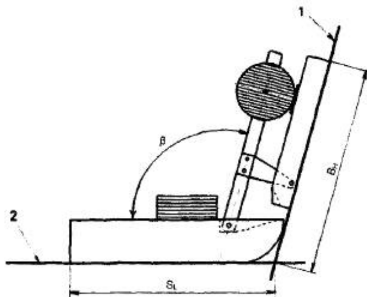
1 — базовая плоскость спинки; 2 — базовая плоскость сиденья
