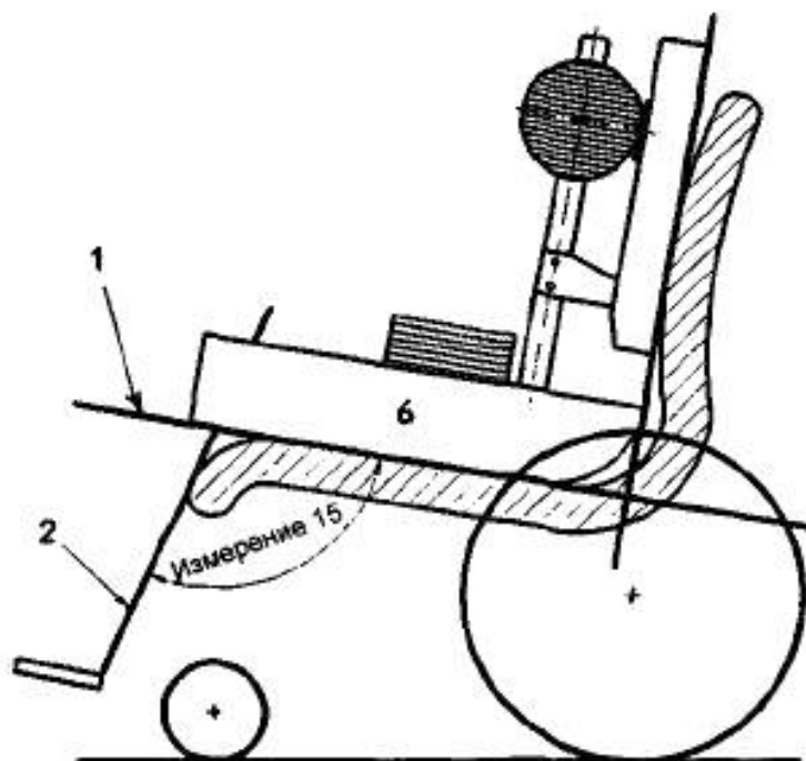
а) Угол наклона подножки к поверхности сиденья
