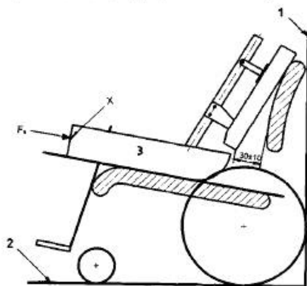
1 — стена; 2 — испытательная площадка; 3 — ЭНУ
