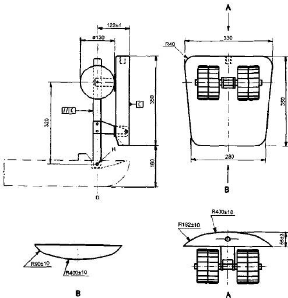
Рисунок А.2 — Узел спинки ЭНУВ
