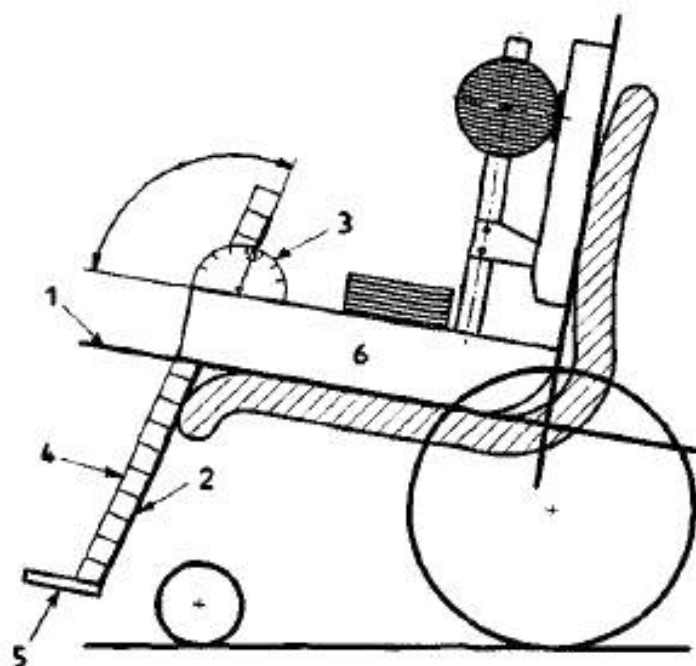
1 — базовая поверхность сиденья; 2 — базовая поверхность подножки; 3 — средства измерения углов; 4 — стальная планка; 5 — опора стопы; 6 — ЗНУ
