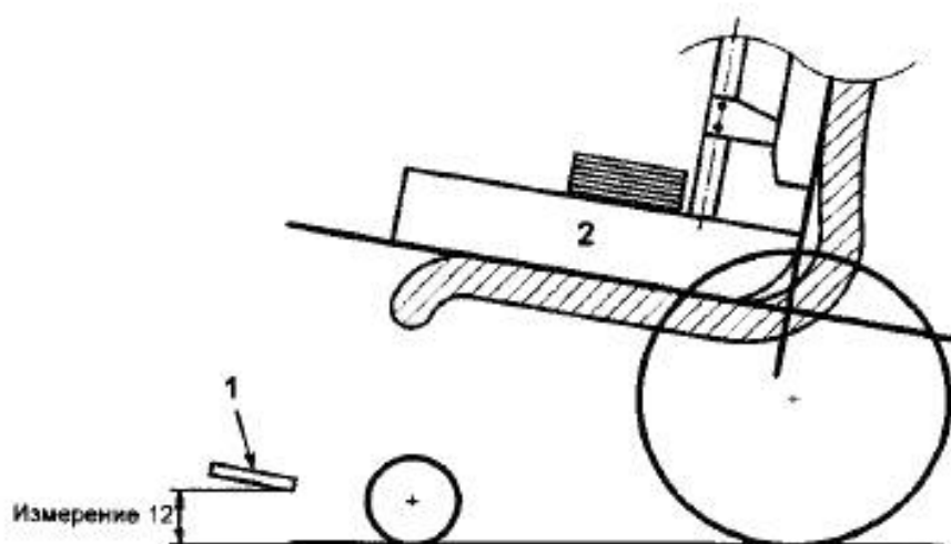
Рисунок 21 — Клиренс опоры стопы
