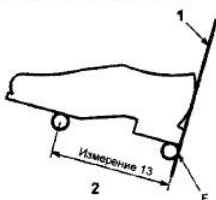
а) Длина опоры стопы трубчатой формы
