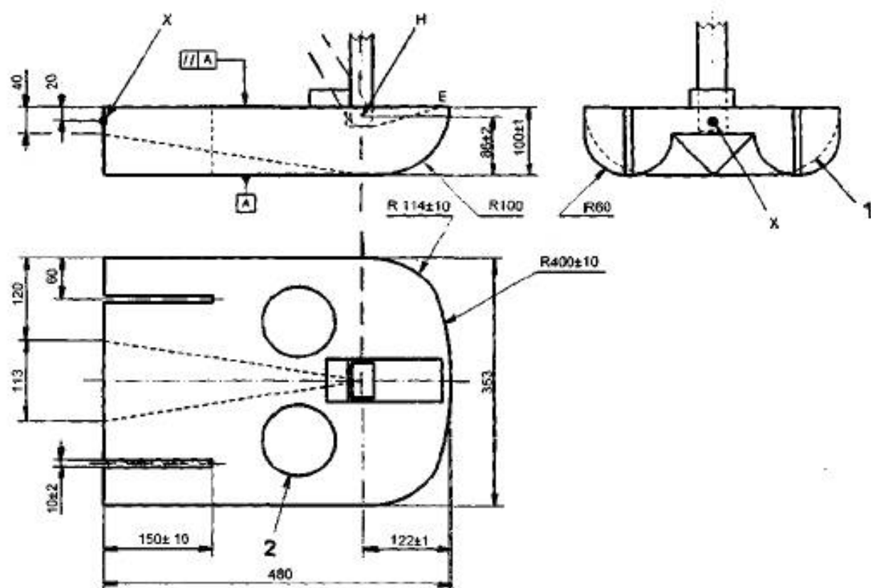
Рисунок А.1 — Узел сиденья ЭНУВ
