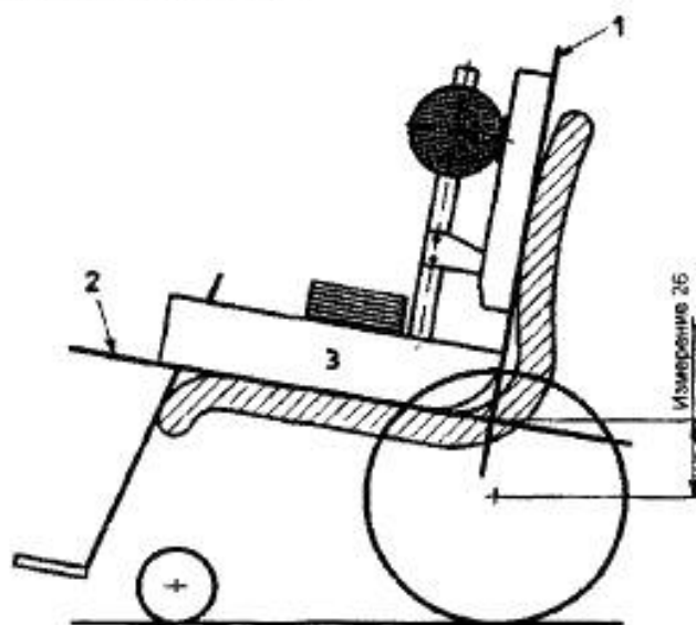
Рисунок 35 — Вертикальное положение оси ведущего колеса
