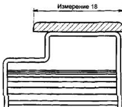
Рисунок 27 — Длина подлокотника
