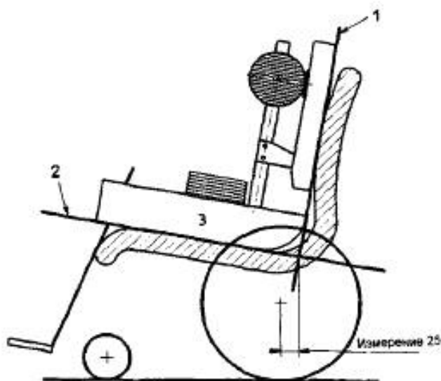
а) Горизонтальное положение оси ведущего колеса
