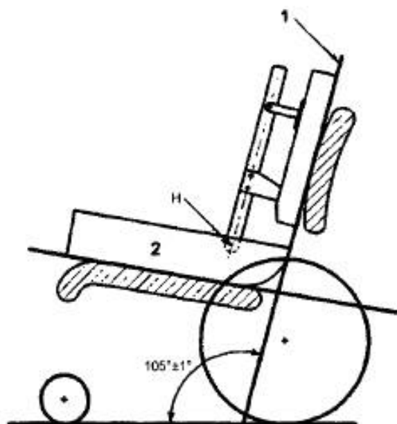
1 — базовая плоскость спинки; 2 — ЭНУ
