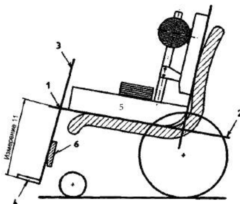
Рисунок 20 — Длина подножки
