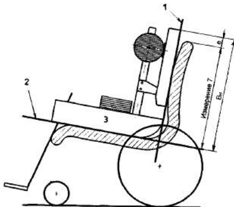
1 — базовая плоскость спинки; 2 — базовая плоскость сиденья; 3 — ЭНУ
