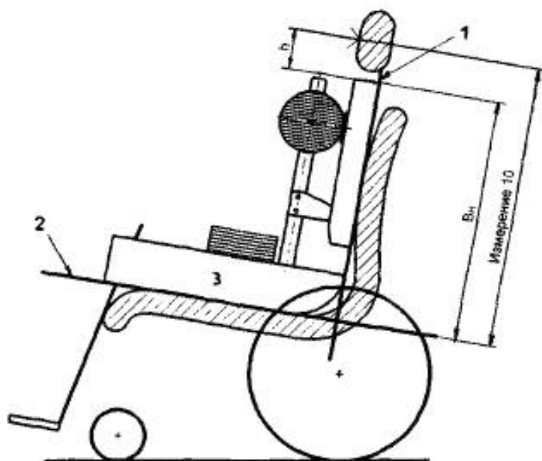
Рисунок 19 — Высота подголовника над сиденьем
