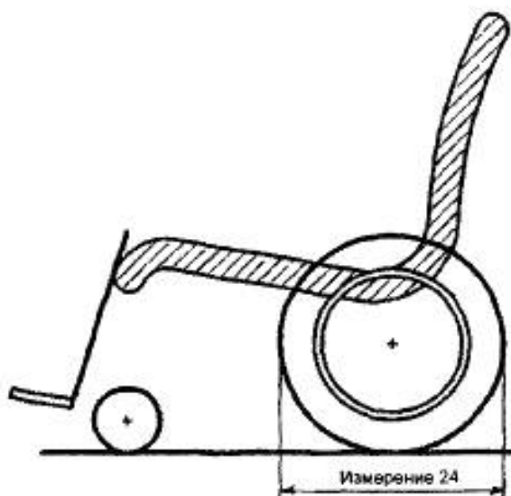
Рисунок 33 — Диаметр ведущего колеса
