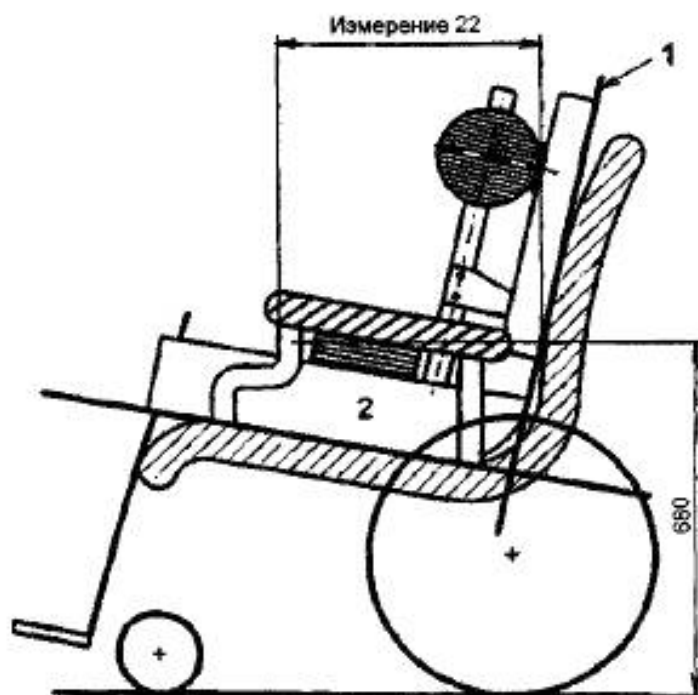
Рисунок 31 — Расположение подлокотника
