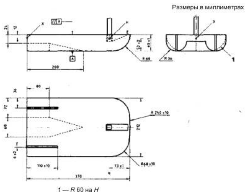
Рисунок А.4 — Узел сиденья ЭНУВ
