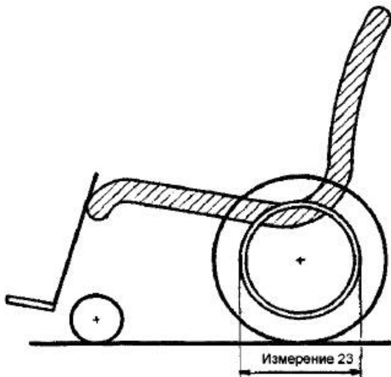
Рисунок 32 — Диаметр обода ручного привода
