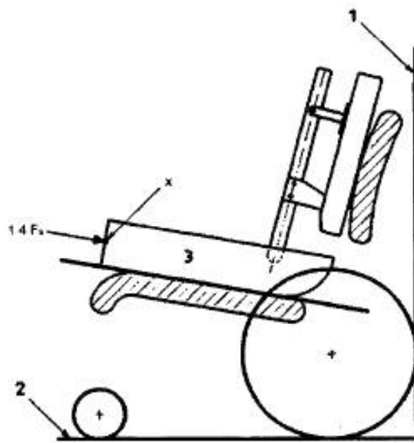
1 — стена; 2 — испытательная площадка; 3 — ЭНУ
