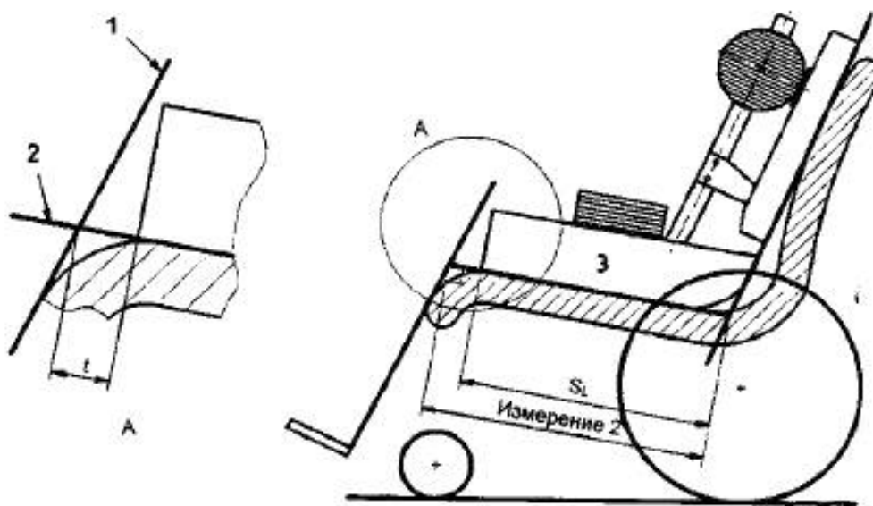
1 — базовая плоскость подножки; 2 — базовая плоскость сиденья; 3 — ЭНУ
