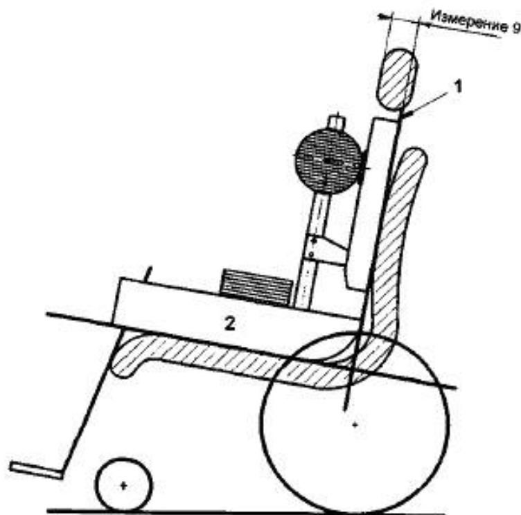
1 — базовая плоскость спинки; 2 — ЗНУ
