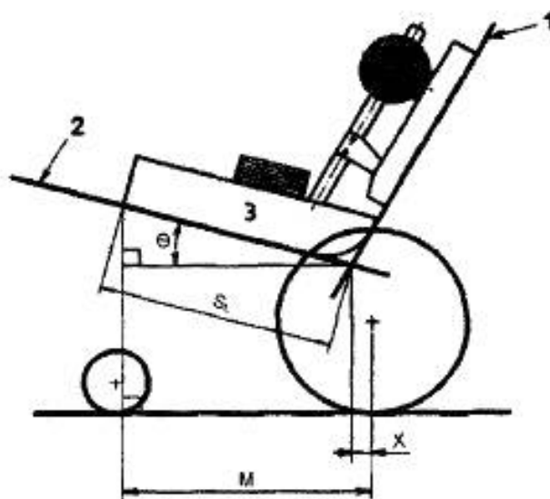
1 — базовая плоскость спинки; 2 — базовая плоскость сиденья; 3 — ЗНУ
