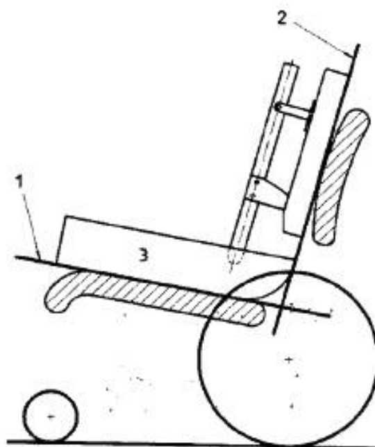
1 — базовая плоскость сиденья; 2 — базовая плоскость спинки; 3 — ЭНУ
