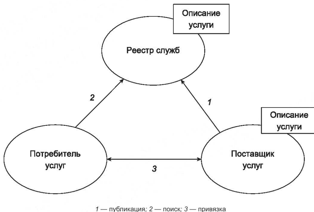
Рисунок 1 — Основные роли в SOA
