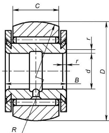
Рисунок 5 — Конструктивные исполнения 91К1, 91Ю2
