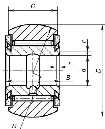
Рисунок 6 — Конструктивные исполнения 91К2, 91Ю3
