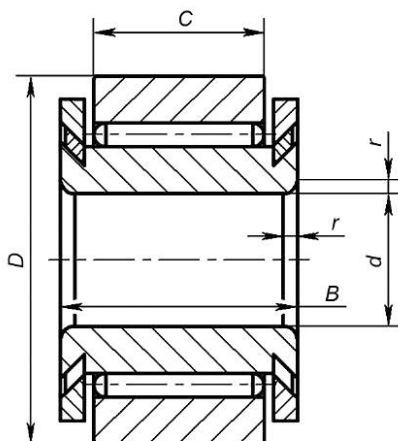
Рисунок 3 — Конструктивные исполнения 91, 91Ю
