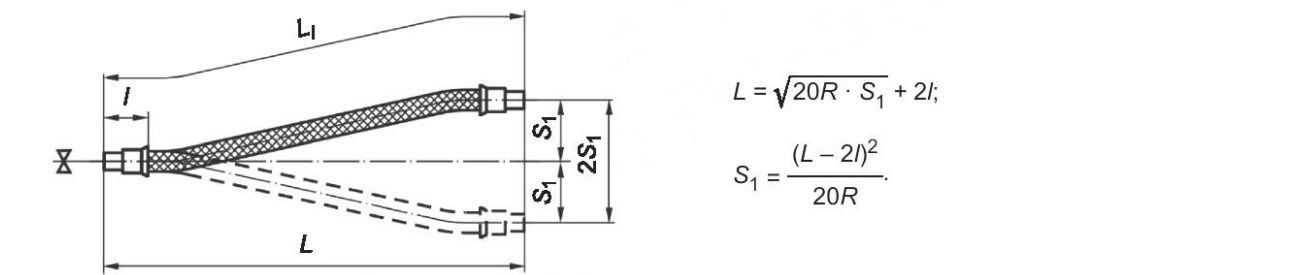
Рисунок Д.3 — Схема монтажа для компенсации перемещения конца шланга в направлении, перпендикулярном к его оси. Установка шлангов для компенсации сдвиговых перемещений (без вибрации)
