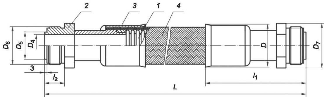
1 — гофрированная труба; 2 — наконечник; 3 — втулка; 4 — оплетка
