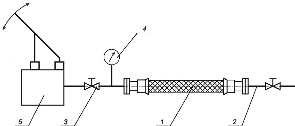
Рисунок Г.1 — Испытания шланга на прочность
