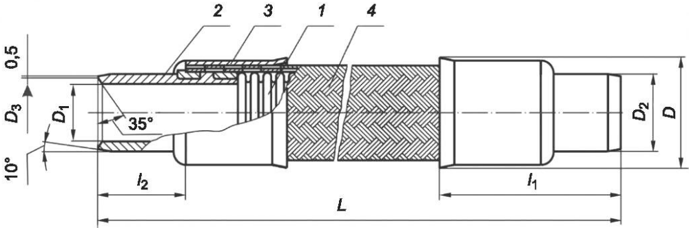
1 — гофрированная труба; 2 — наконечник; 3 — втулка; 4 — оплетка
