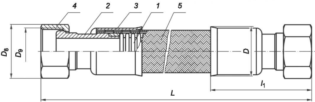
1 — гофрированная труба; 2 — ниппель; 3 — втулка; 4 — накидная гайка; 5 — оплетка
