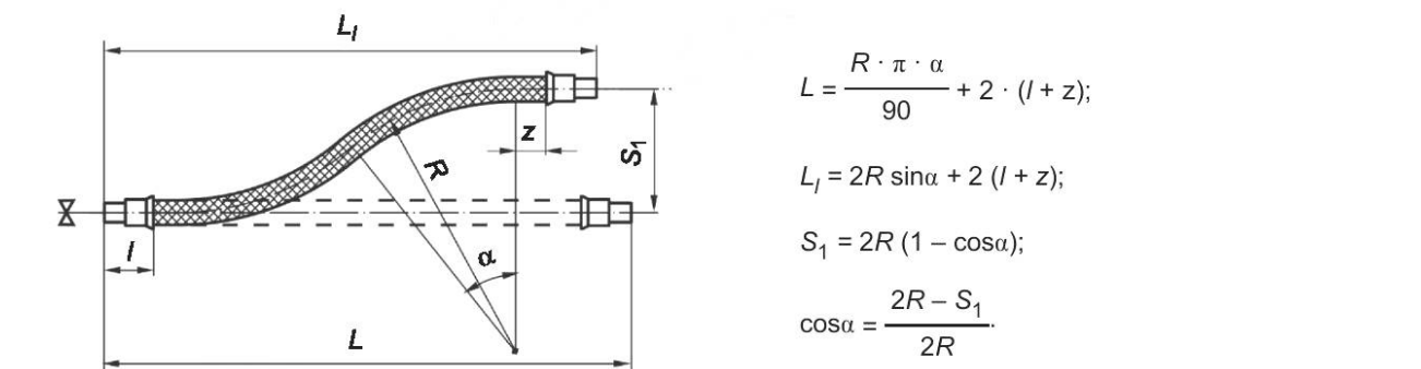
Рисунок Д.2 — Схема монтажа для компенсации перемещения конца шланга в направлении, перпендикулярном к его оси
