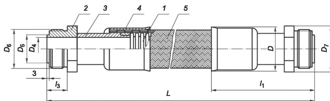
1 — гофрированная труба; 2 — штуцер; 3 — наконечник; 4 — втулка; 5 — оплетка
