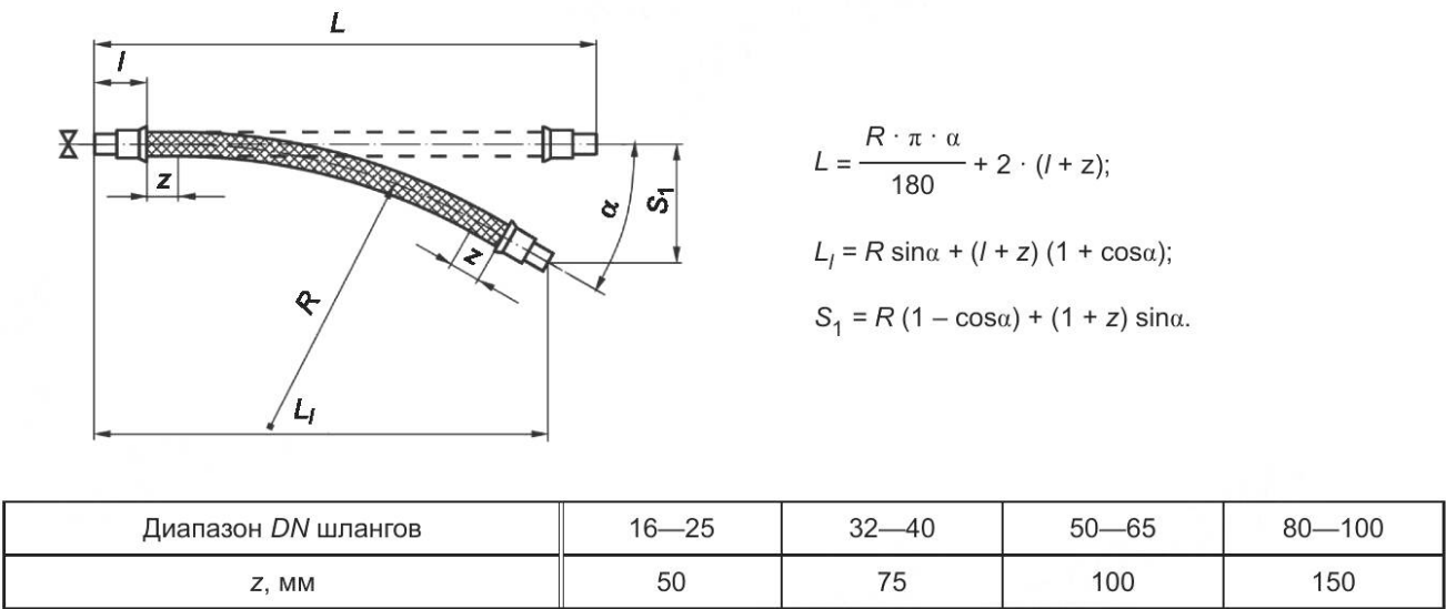
Рисунок Д.1 — Схема монтажа для компенсации угловых перемещений
