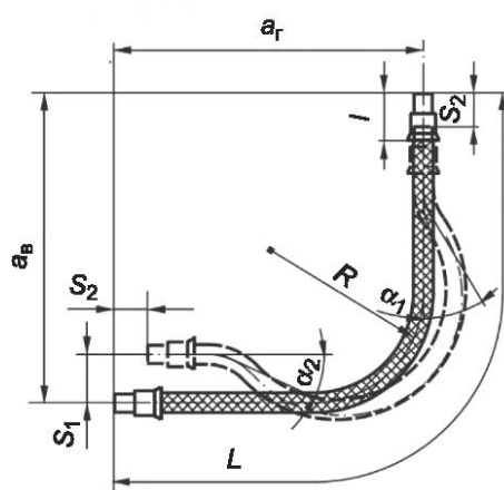
Рисунок Д.9 — Схема монтажа для компенсации перемещения конца шланга одновременно в двух направлениях (перпендикулярном и вдоль его оси) при малой частоте перемещения (без вибрации)
