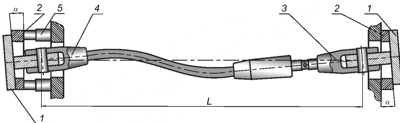
1 — плита с проушиной (не входит в состав образца); 2 — клиновая плита; 3 — регулируемая вилка; 4 — нерегулируемая вилка; 5 — привод осевого перемещения; \alpha = 0,6^\circ или 10 мрад; L \geq 5 м
