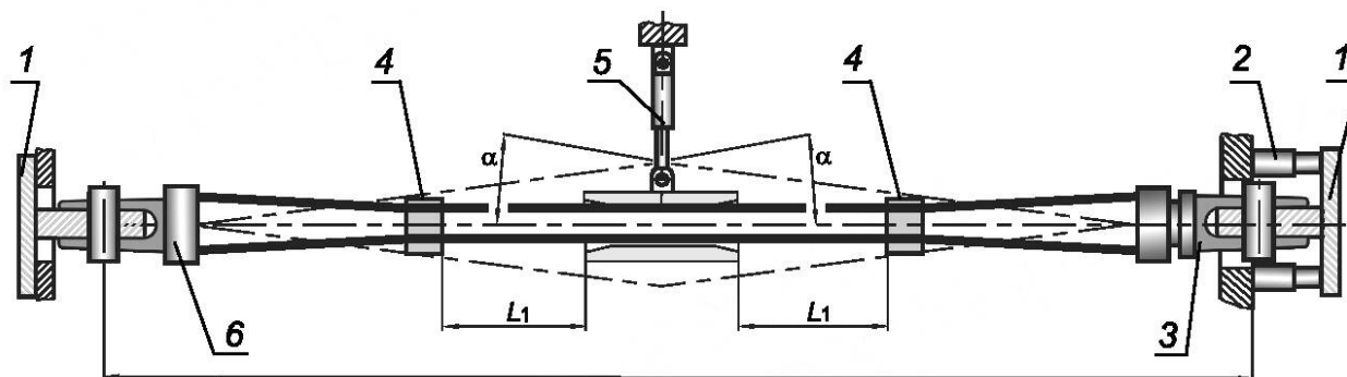
1 — плита с проушиной (не входит в состав образца); 2 — привод осевого перемещения; 3 — регулируемая вилка; 4 — свободный девиатор; 5 — привод поперечного перемещения; 6 — нерегулируемая вилка; \alpha — см. пункт Б.5; L_1 \geq 0,5 м; L_2 \geq 3,5 м
