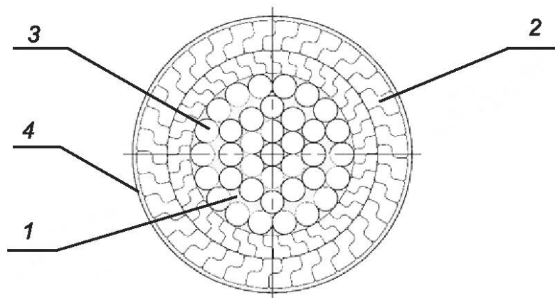
1 — защитная смазка; 2 — зетобразная проволока; 3 — круглая проволока; 4 — оболочка
