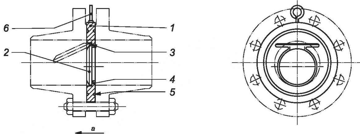
1 — корпус; 2 — клапан; 3 — шпилька; 4 — уплотнение клапана; 5 — уплотнение корпуса; 6 — подъемная петля; a — направление потока рабочей среды
