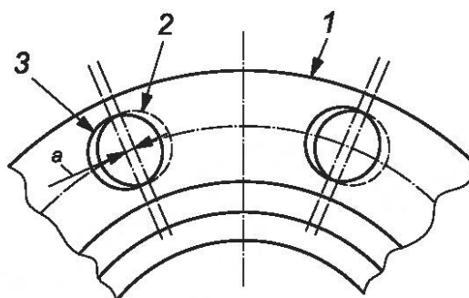
1 — фланец; 2 — отверстия в первом фланце; 3 — отверстия в противоположном фланце для выравнивания; а — смещение отверстия под болт (см. 6.10.1.4)
