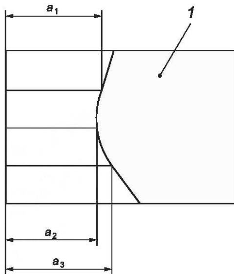
Рисунок 3 — Определение общей длины трещины по поверхности разрушения
