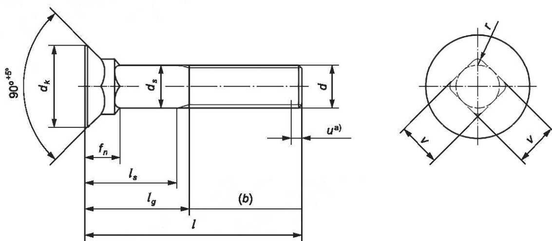
Рисунок 1 — Болт с потайной головкой и низким квадратным подголовком
