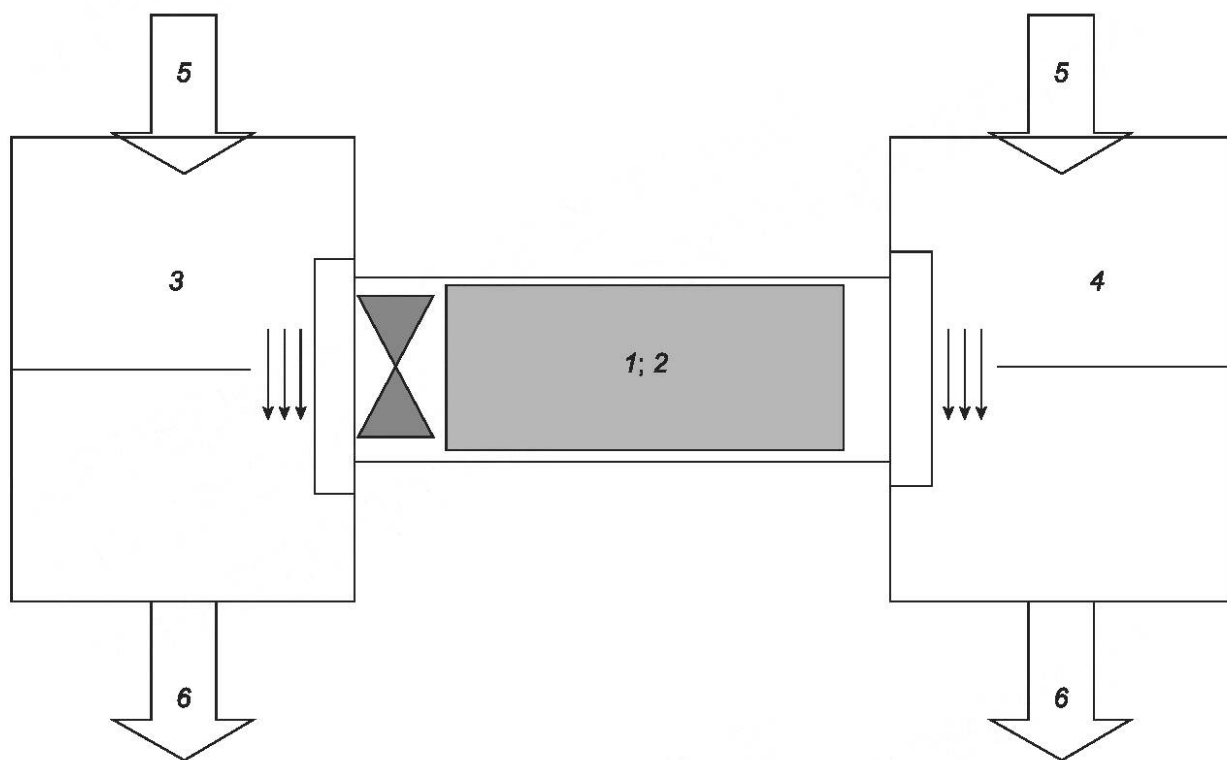
1 — устройство 1; 2 — устройство 2; 3 — внутренняя камера; 4 — наружная камера; 5 — распределитель воздуха; 6 — воздухозаборник; \downarrow\downarrow\downarrow — скорость продувочного воздуха более 0,05 \text{ м/с}
