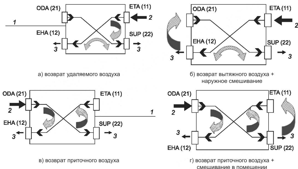
Рисунок 1 — Схематическая конфигурация испытаний на внутренние утечки и смешивание
