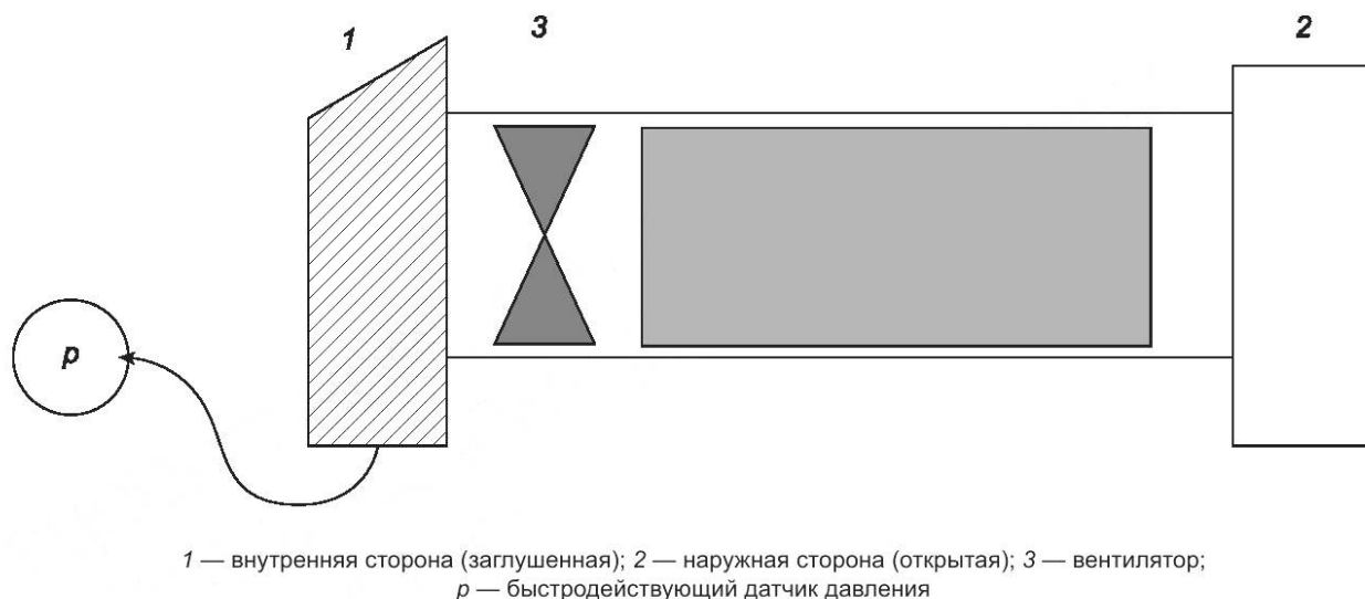
Рисунок 3 — Испытательная конфигурация для измерения давления
