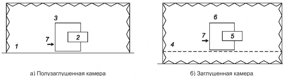
1 — полузаглушенная камера; 2 — испытуемый агрегат; 3 — звукопоглощающий и звукоизоляционный кожух; 4 — заглушенная камера; 5 — испытуемый агрегат; 6 — звукопоглощающий и звукоизоляционный кожух; 7 — входящий воздух
