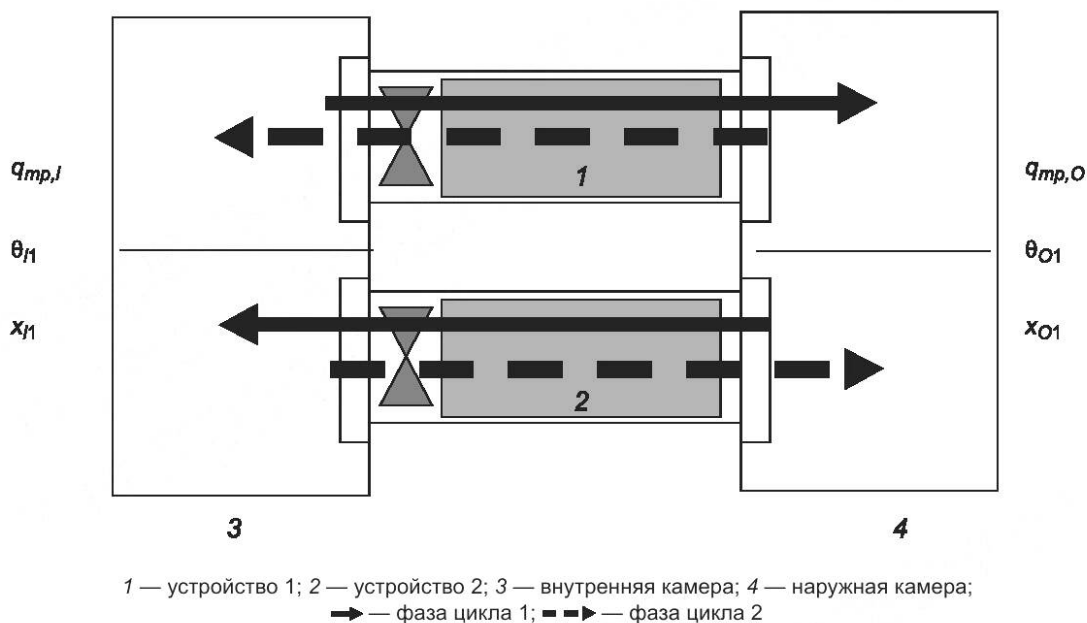
Рисунок 5 — Схема испытательной установки (вид сверху)
