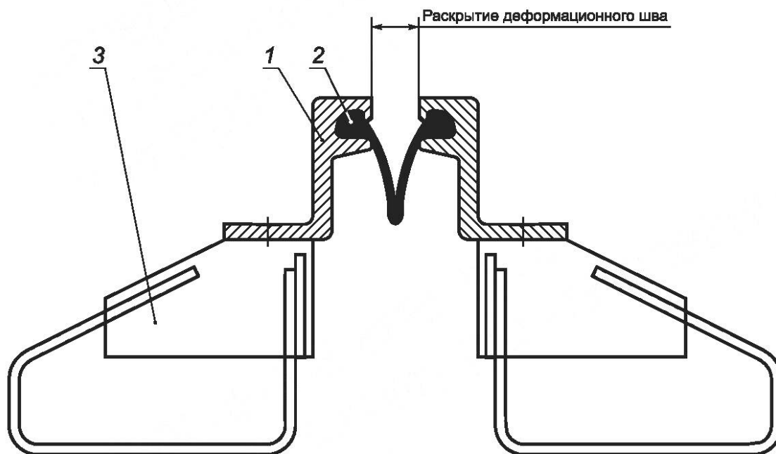
1 — балка окаймления; 2 — компенсатор; 3 — анкерная система
