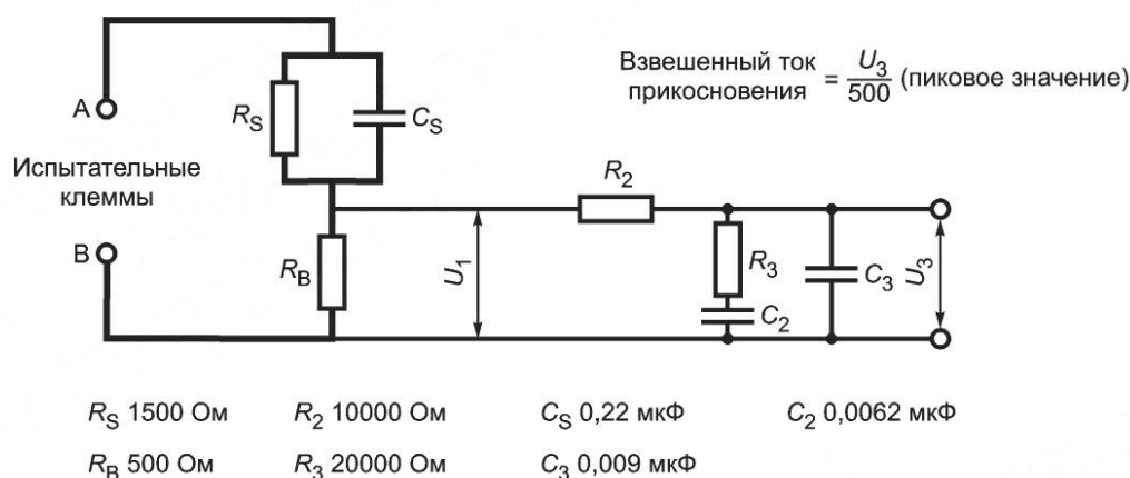
Рисунок 3 — Схема для измерения тока прикосновения \Sigma(I_A)
