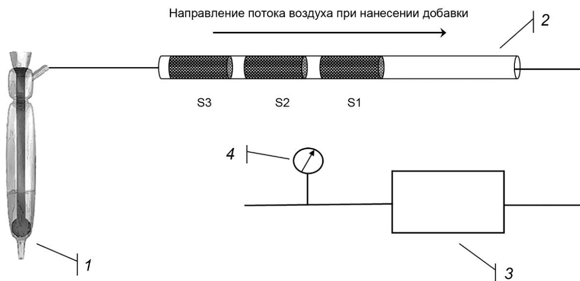
1 — барботер; 2 — сорбционная трубка; 3 — побудитель расхода; 4 — регулятор расхода Рисунок А.4 — Схема внесения добавки на контрольную секцию S3 сорбционной трубки
