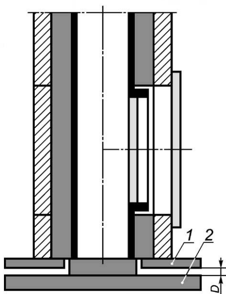
Рисунок А. 5 — Стенд для испытания относительного смещения
