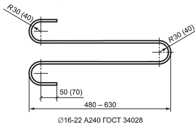
Рисунок Б.4 — Монтажная петля
