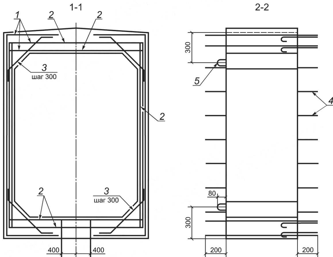
Рисунок Б.1 — Положение арматурного каркаса в звене с приваренными выпусками и монтажными петлями
