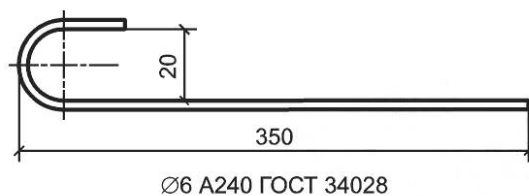
Рисунок Б.3 — Арматурный выпуск
