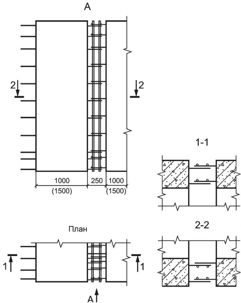
Рисунок А.2 — Стык между звеньями
