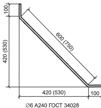
Рисунок Б.2 — Угловой хомут
