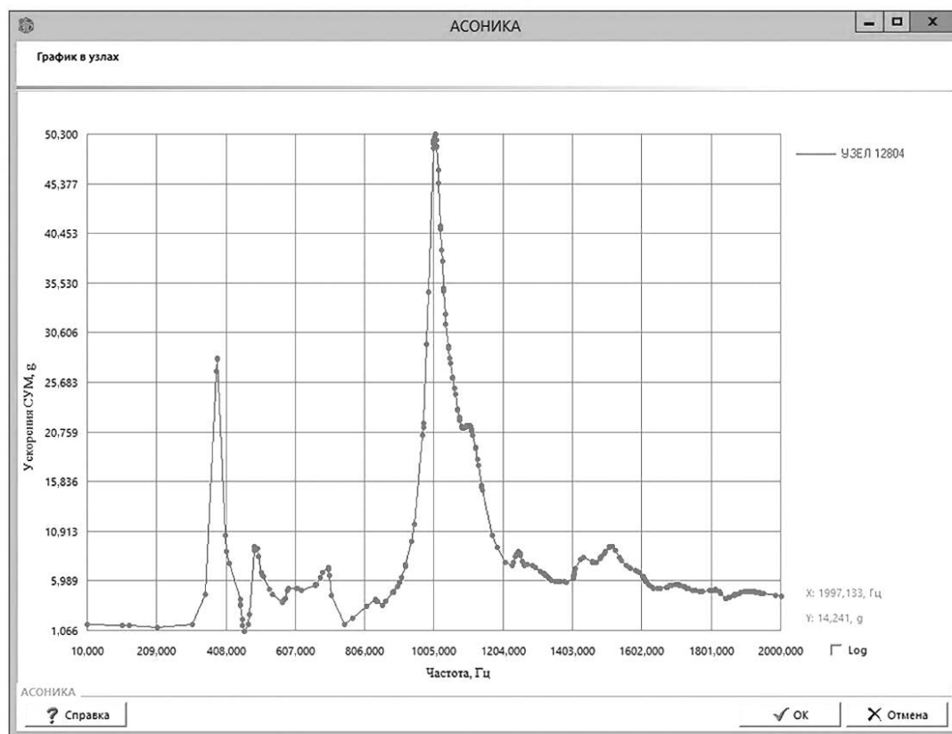
Рисунок А.10 — График зависимости амплитуды суммарного выходного ускорения синусоидальной вибрации от частоты в контрольной точке
