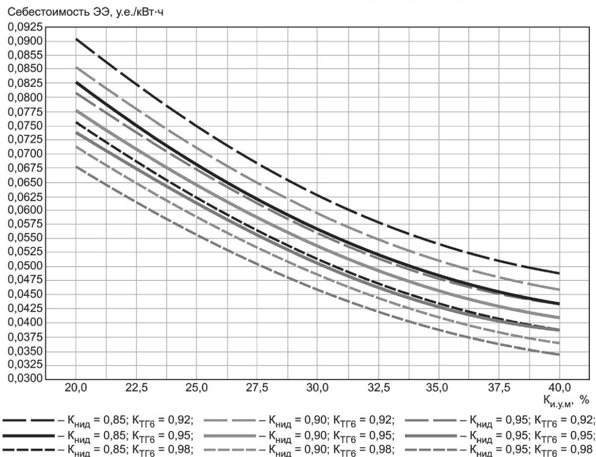
Рисунок 15.6 — Значения C_{ЭЭ} при разных параметрах K_{нид} , K_{ТГ(6)} при K3_{уд} = 2000 у.е./кВт·ч
