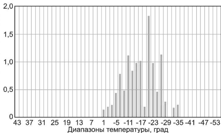
Рисунок 7.8 — Распределение буревых скоростей ветра по градациям температуры на МС в Тикси
