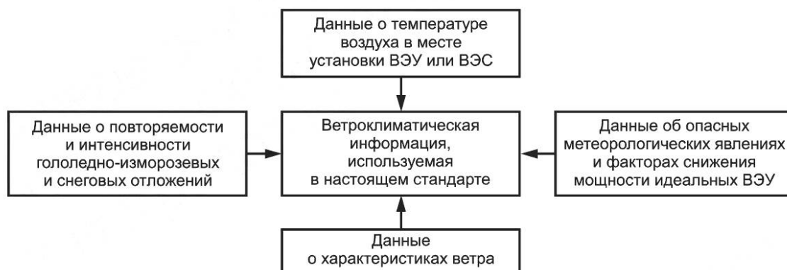
Рисунок 5.1 — Состав информации, определяющей ВКУ функционирования ВЭУ, ВЭС и ВДЭК и используемой в настоящем стандарте
