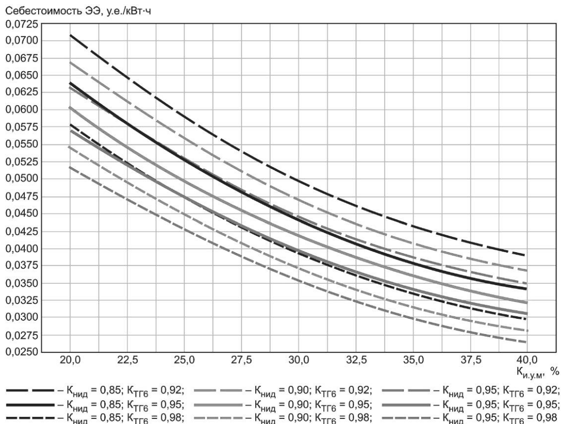
Рисунок 15.5 — Значения C_{ЭЭ} при разных параметрах K_{нид} , K_{ТГ(6)} при K3_{уд} = 1500 у.е./кВт·ч
