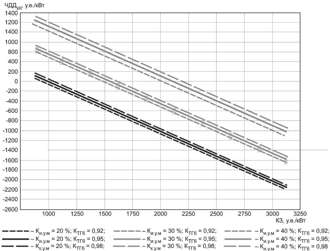
Рисунок 15.8 — Зависимость удельного дисконтированного дохода ЧДД уд от параметров КЗ, К и.у.м , К ТГ(6) для значений К нид = 0,95 и К ТГ = 0,95
