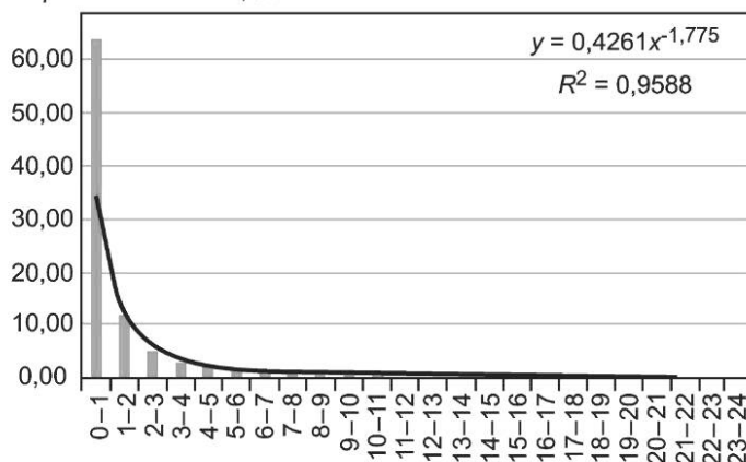
Рисунок 7.6 — Плотность вероятности штилей на МС в Тикси
