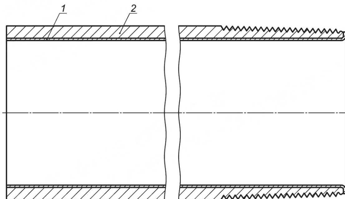
1 — лейнер; 2 — НКТ
