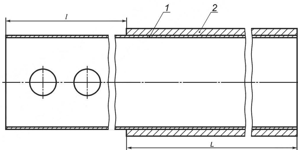
1 — лейнер; 2 — НКТ
