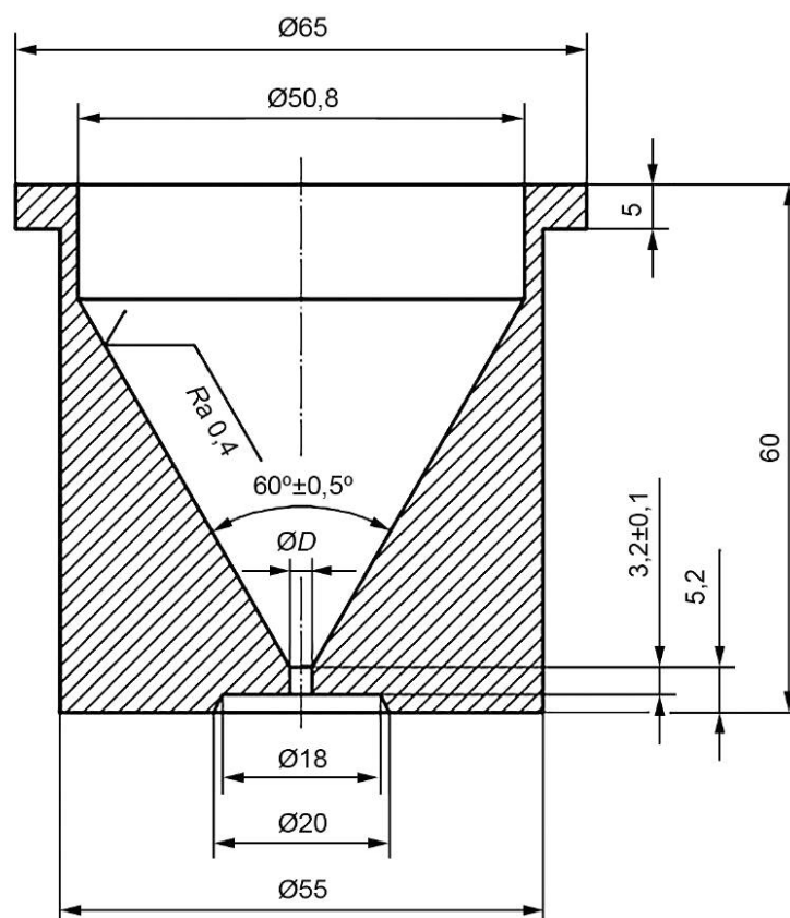
Рисунок 1 — Воронка Холла
