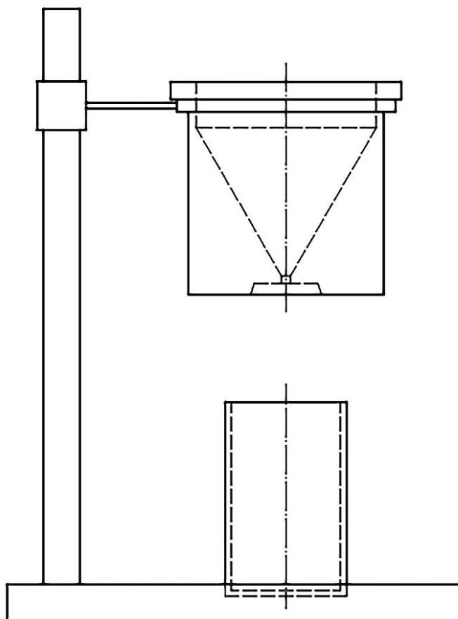
Рисунок 2 — Схема установки воронки на стойке
